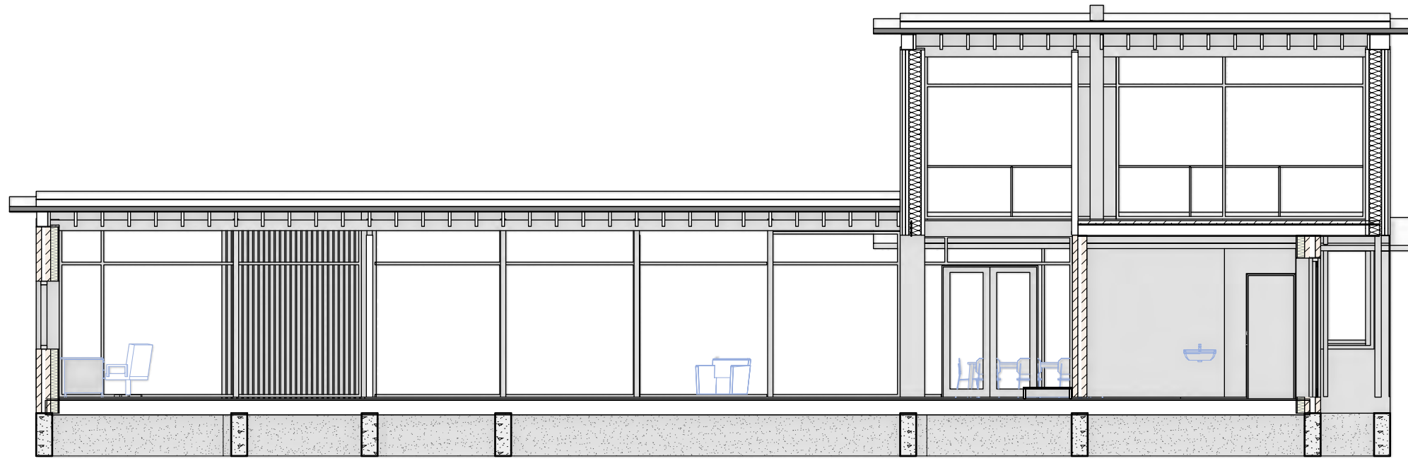
Doorsnede AA'
