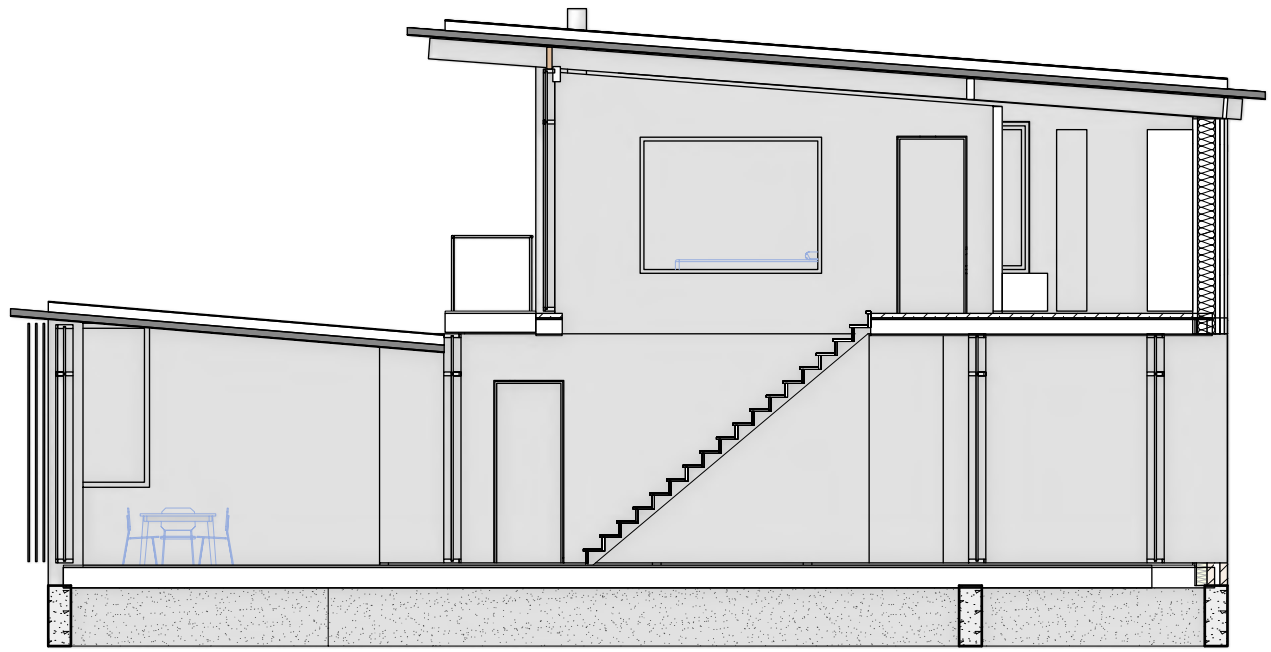
Doorsnede BB'
