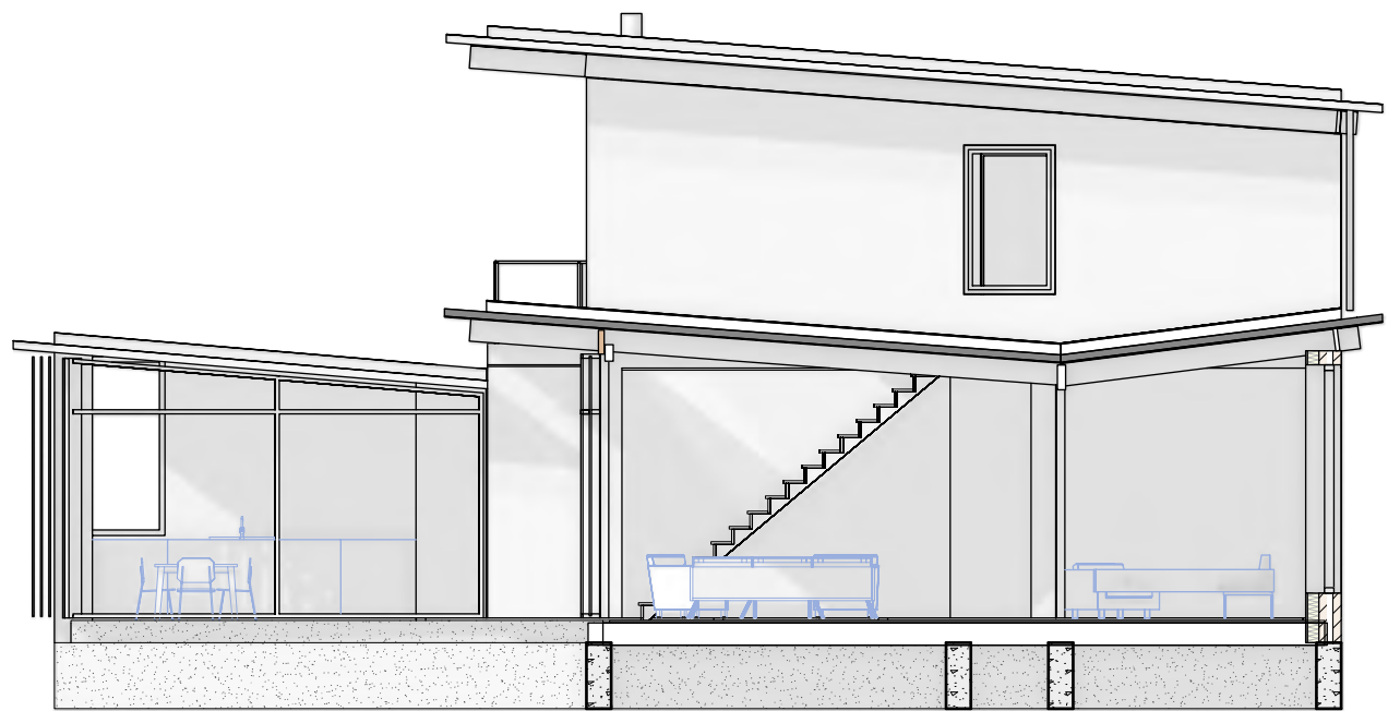
Doorsnede CC'
