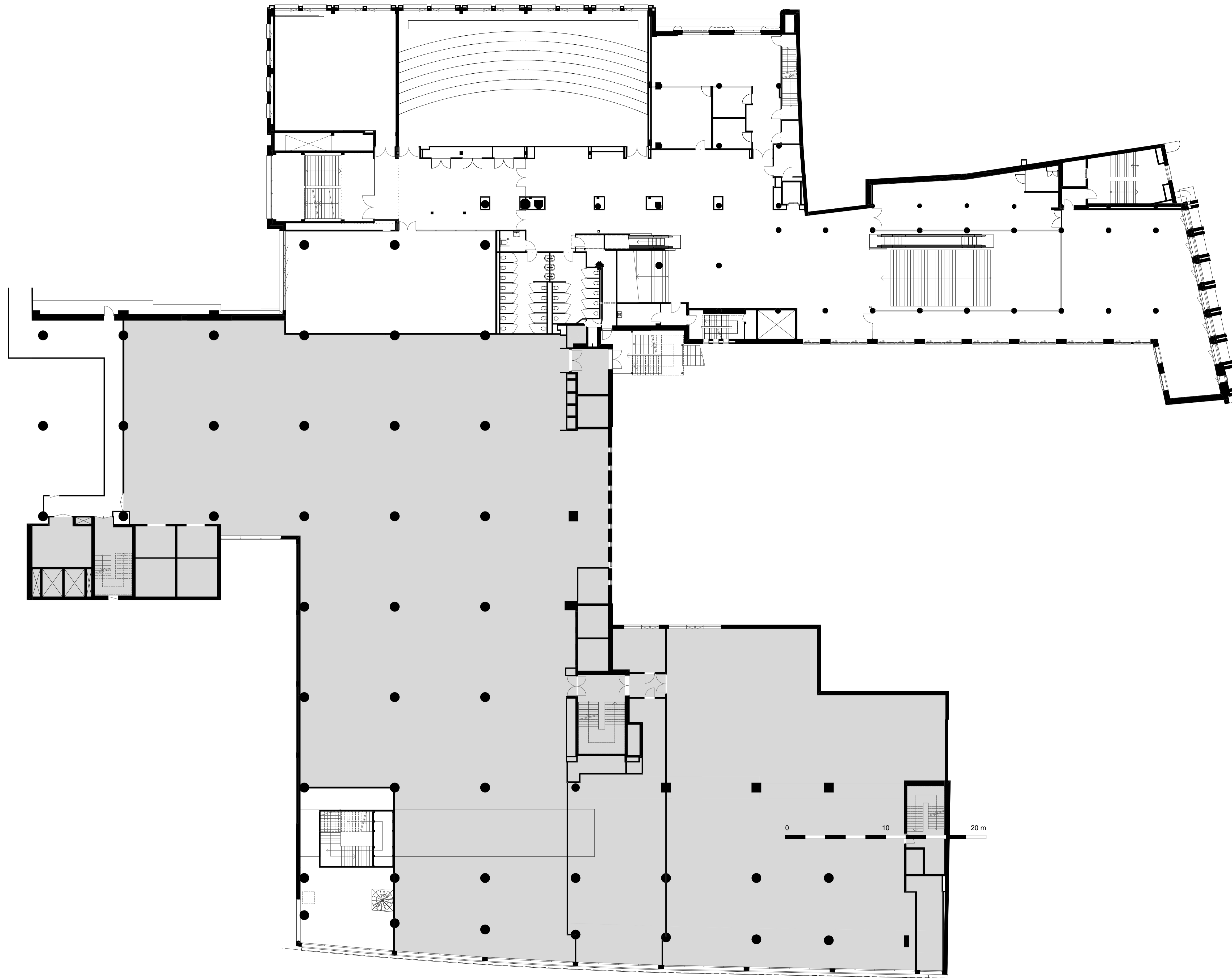
Plattegrond 1e verdieping
