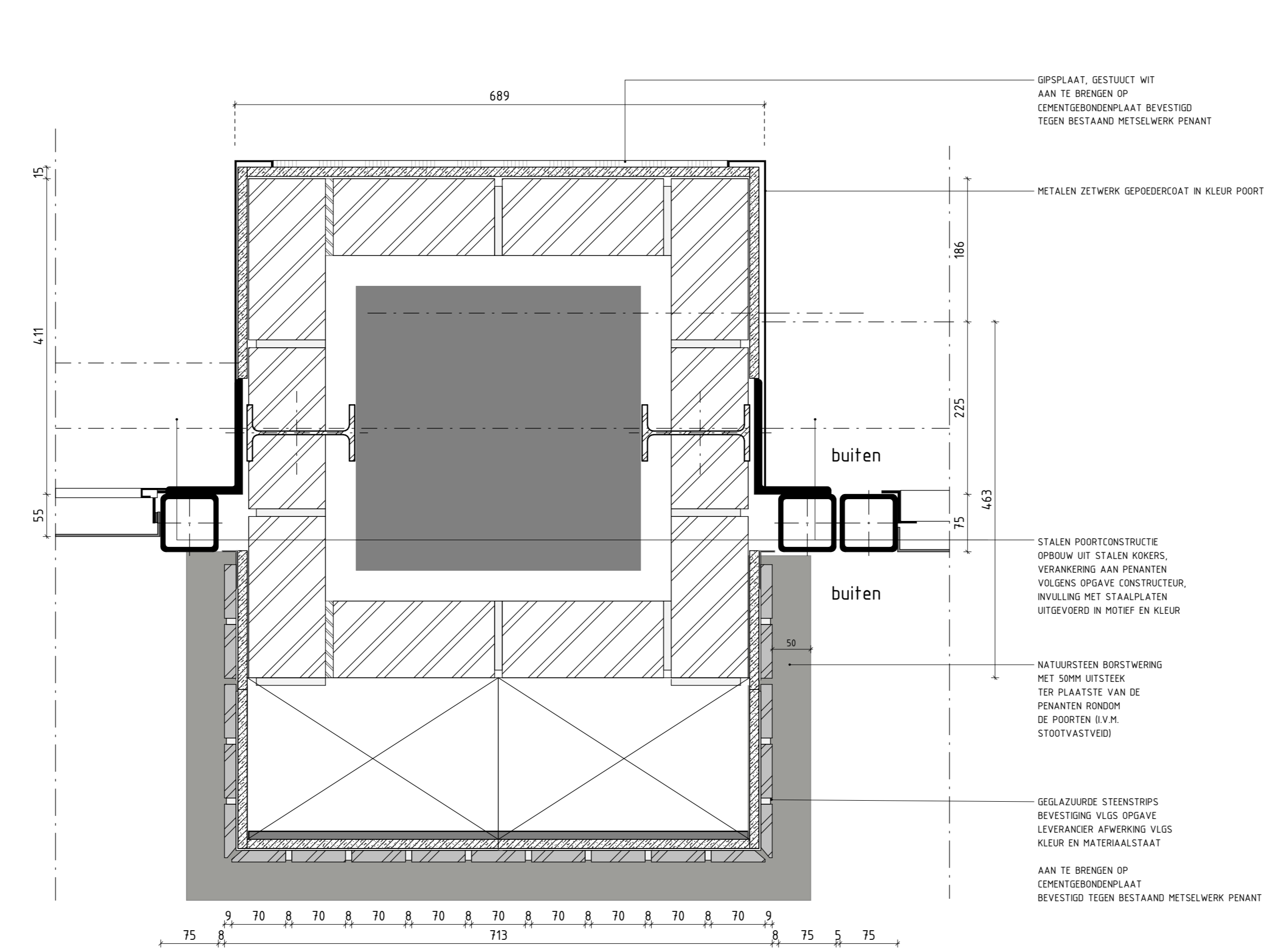
horizontaal detail middenpenant schaal 1:5
