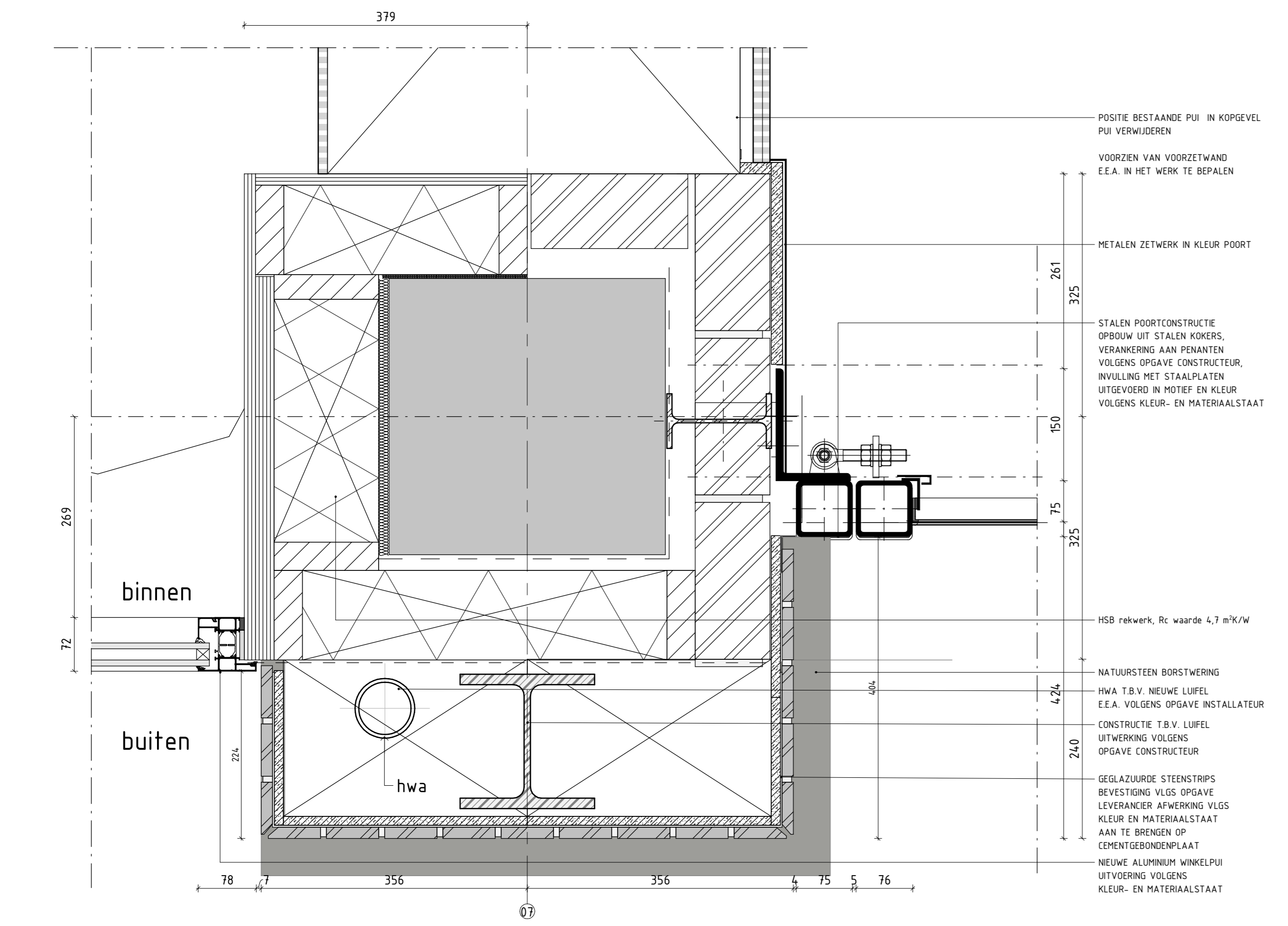
horizontaal detail linker/rechter penant schaal 1:5
