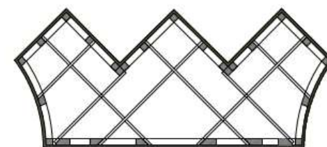
hor. doorsnede podiumdeel C
