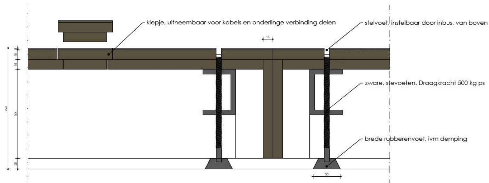
hor. doorsnede podiumdeel A / A'
