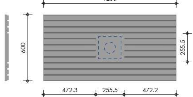
M special M - opliggend vlak groot - hart tbv spot / rookmelder / speaker / ... 1200 x 600 Troldekt® line
