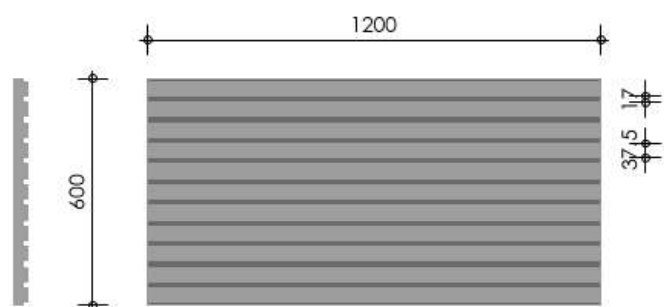
A standaard 1200 x 600 Troldekt® line
