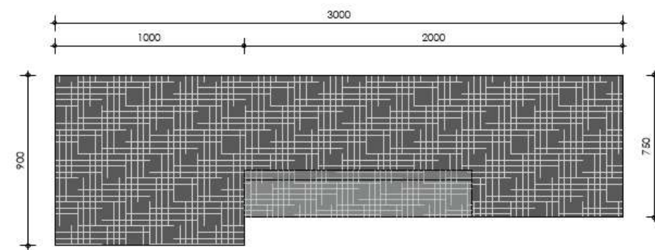
bovenaanzicht korte bank 1:20
