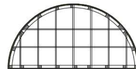
hor. doorsnede podiumdeel D / D'
