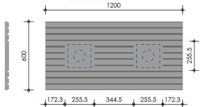
L special L - opliggend vlak groot - dubbel tbv spot / rookmelder / speaker / ... 1200 x 600 Troldekt® line
