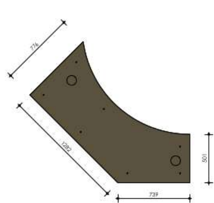
podiumdeel A / A' ( 2x )
