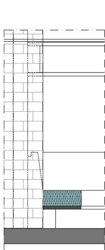
AANZICHT A 1:10
