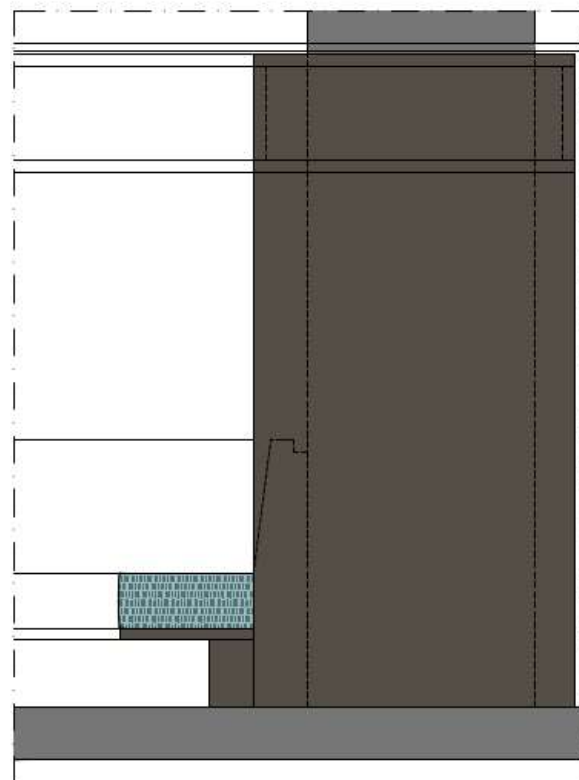
AANZICHT BANK D 1:10
