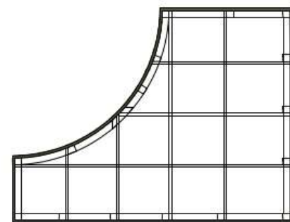
hor. doorsnede podiumdeel B / B'
