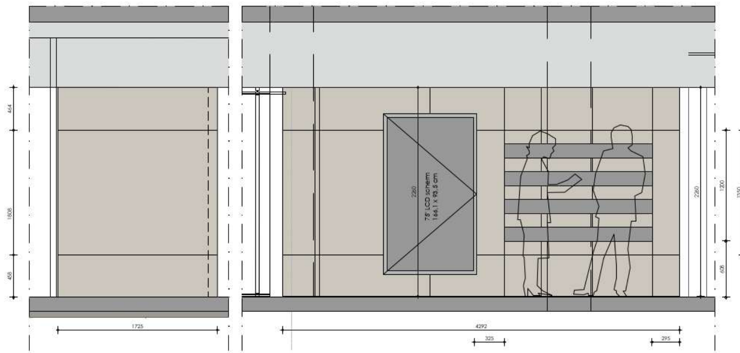
aanzicht A - 1:20
