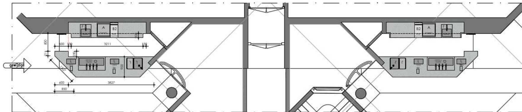
BOVENAANZICHT BLAD 1:50
