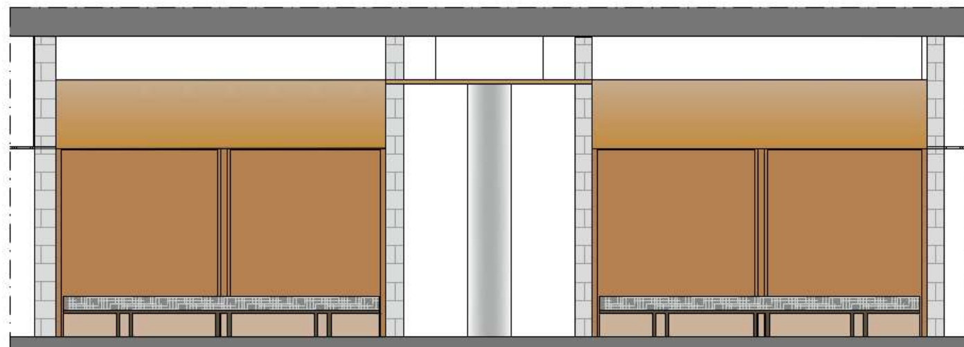
aanzicht banken in nissen 1:20
