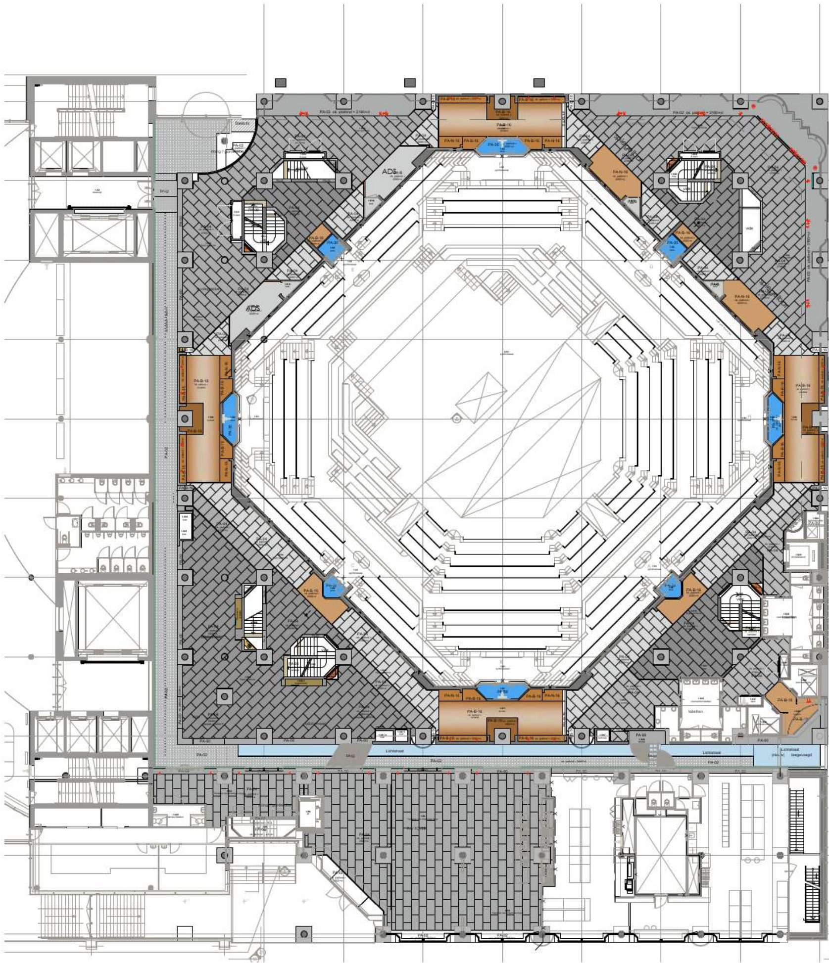
PLAFOND 1e VERDIEPING 1:100
