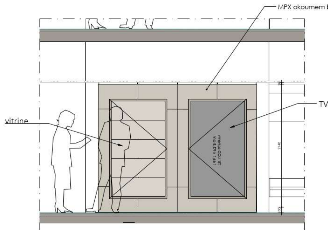
aanzicht voorzetwand met TV en vitrine - beg.gr.ond 1:20 komt 1 x voor
