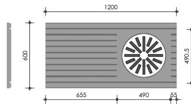
i special i - rooster opliggend 400 rond 1200 x 600 Troldekt® line SPARING Ø 360 mm
