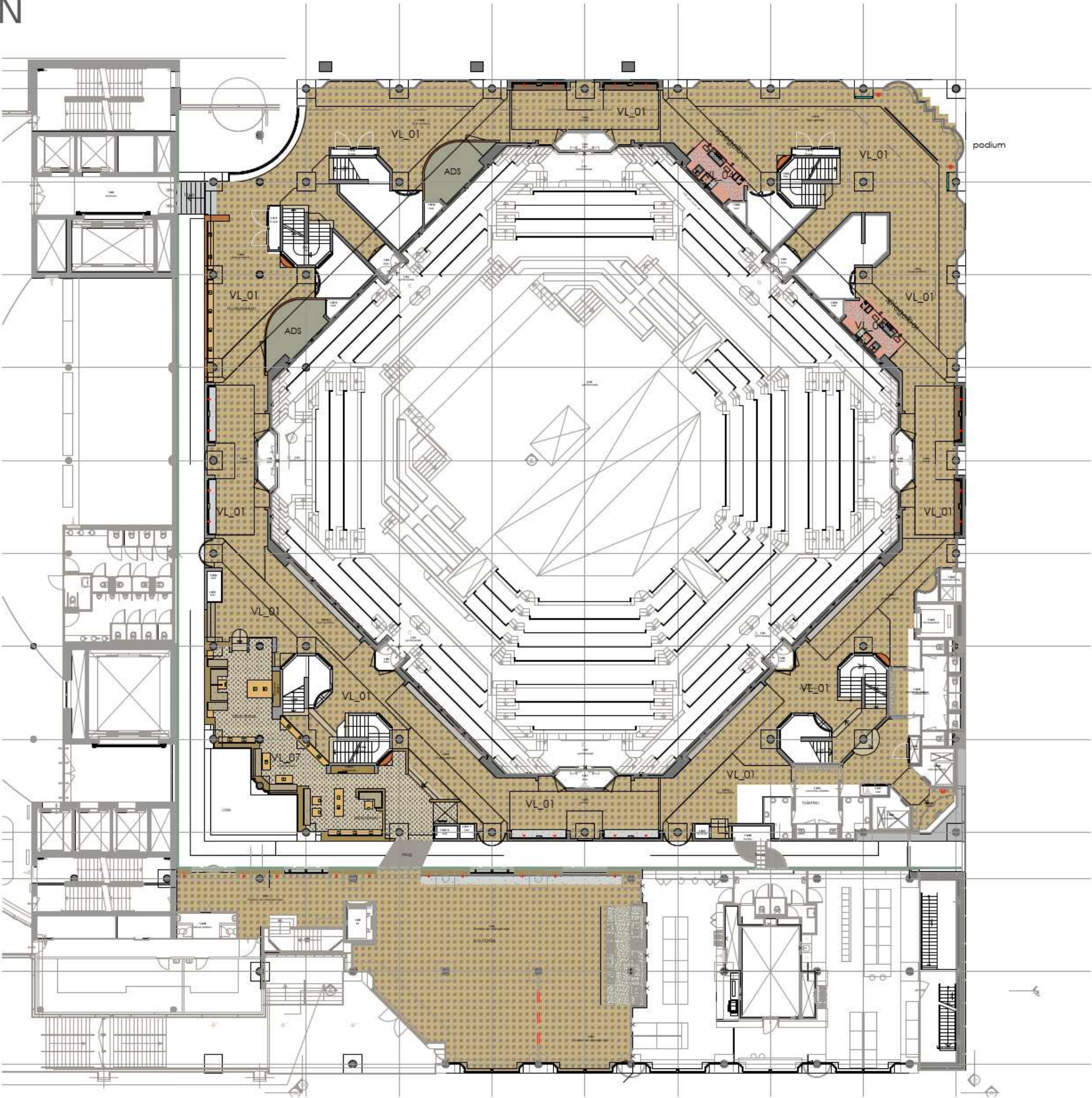
VLOERAFWERKING 1e VERDIEPING 1:100
