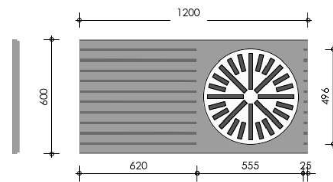
j special j - rooster opliggend 500 rond 1200 x 600 Troldekt® line SPARING Ø 460 MM
