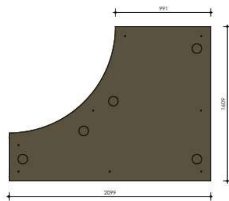
podiumdeel B / B' ( 2x )
