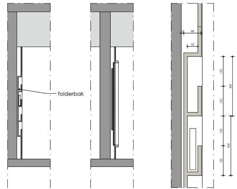
doorsn. D 1:20
