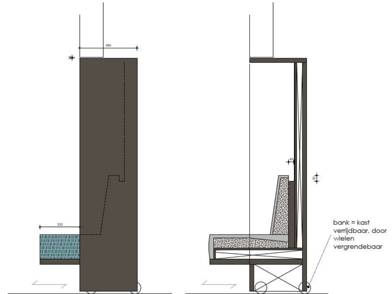
ZIJAAANZICHT BANK 1:20
