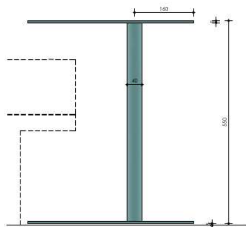
BOVENAANZICHT 1:5
