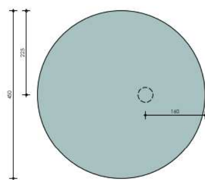
BOVENAANZICHT 1:5
