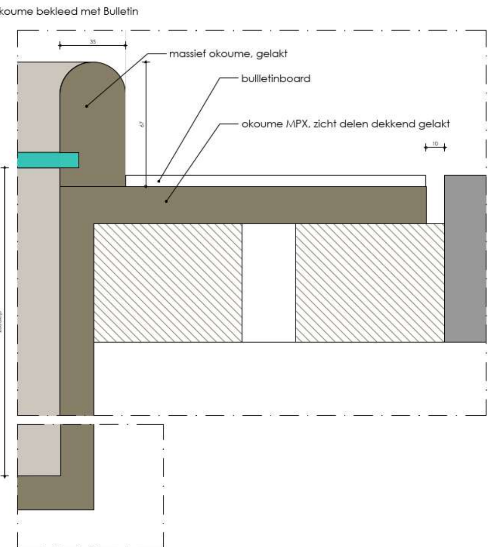
detail A - 1:1 - lijst rondom TV
