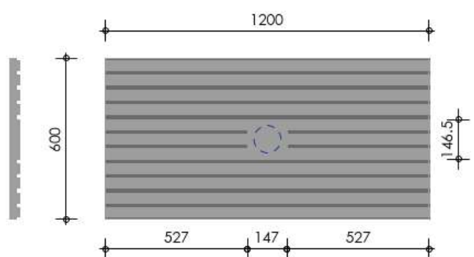
G special G - 1 x spot opliggend - hart plaat 1200 x 600 Troldekt® line
