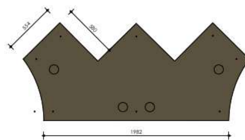
podiumdeel C ( 1x )
