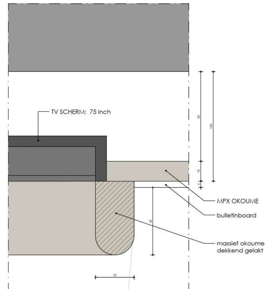
detail 1:1 - lijst rondom TV
