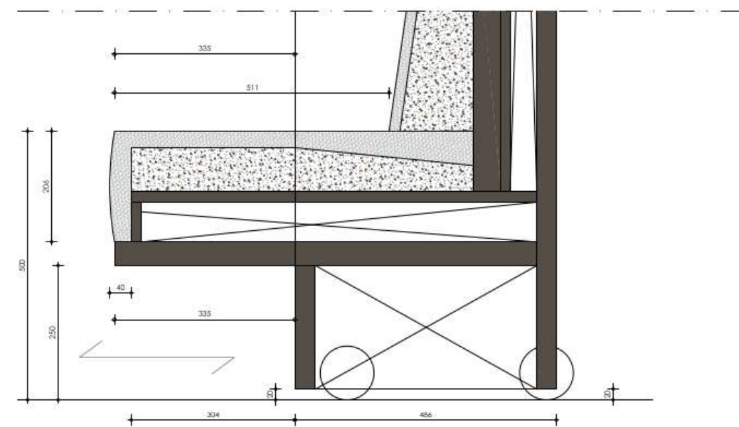
VERT. DOORSNEDE BANK 1:5
