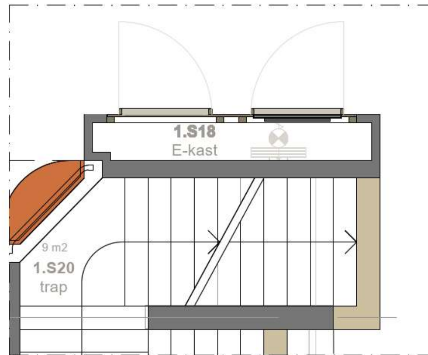
doorsnede voorzetwand met 1 TV + 1 x frame met bulletingboard 1e verdieping 1:20 - komt 3 x voor
