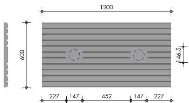
F special F - 2 x spot opliggend 1200 x 600 Troldekt® line
