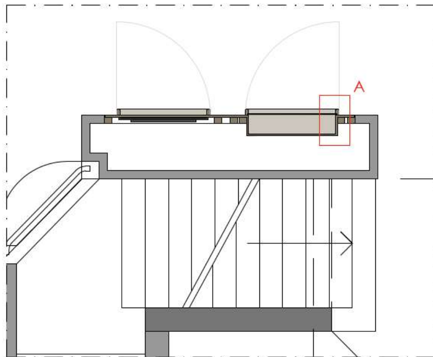
doorsnede voorzetwand met TV en vitrine - beg.gr.ond 1:20 komt 1 voor
