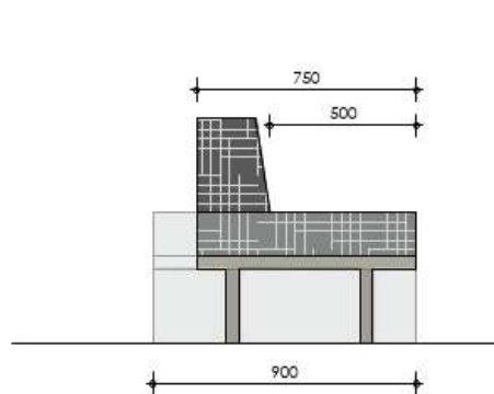
zij aanzicht A :20
