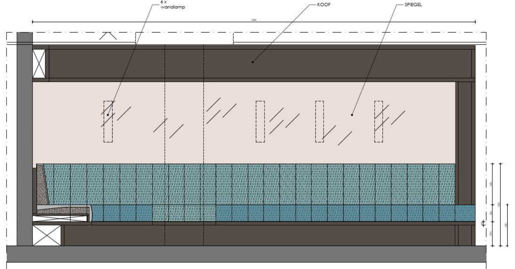
VOORAANZICHT BANK C 1:10
