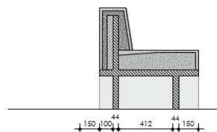
doorsnede C :20
