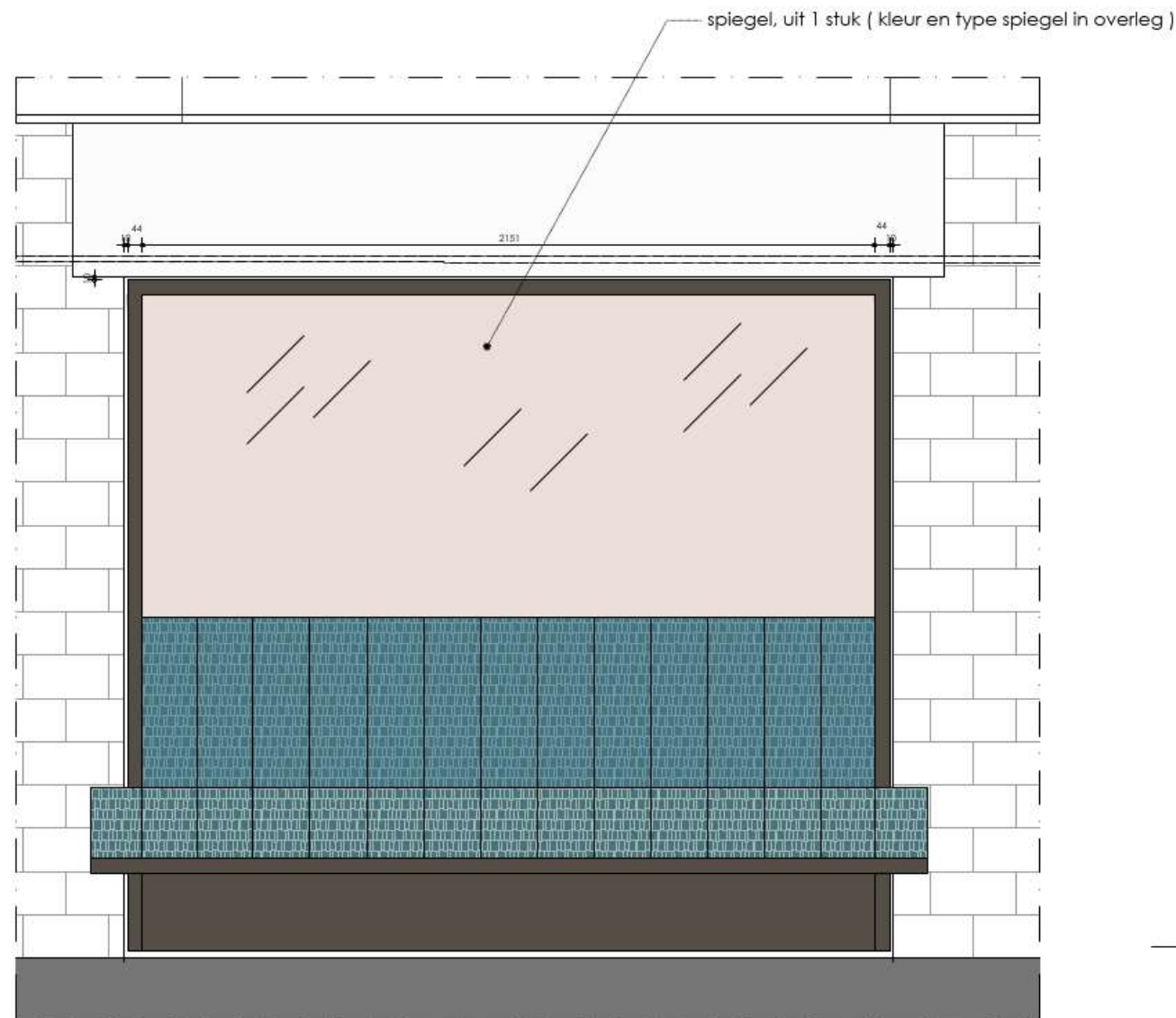
VOORAANZICHT BANK 1:20
