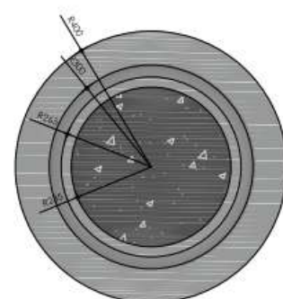
bovenaanzicht rond 1:10 ( 1 stuk )
