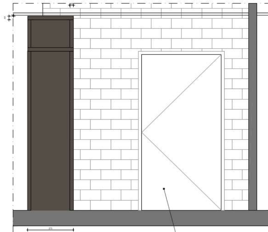
AANZICHT BANK E 1:10
