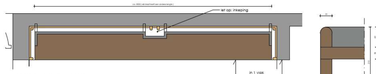
bovenaanzicht blad 1:10
