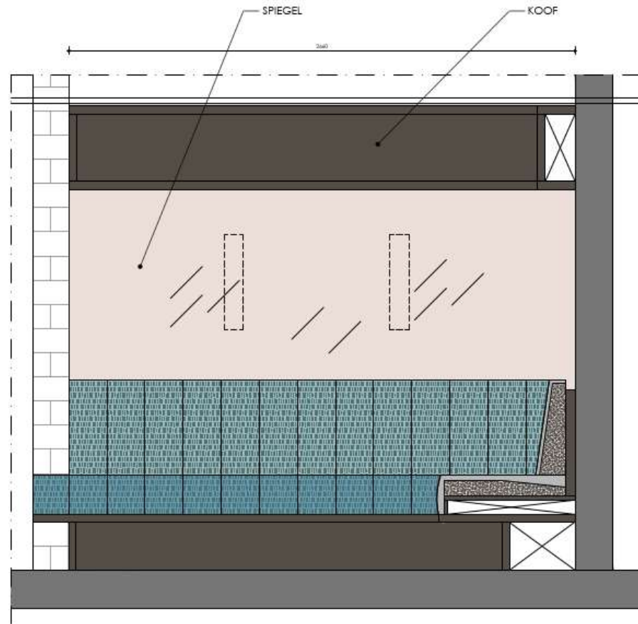
VOORAANZICHT BANK B 1:10
