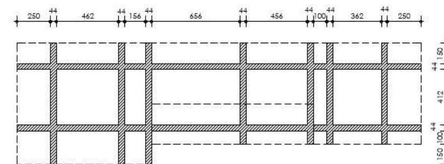
bovenaanzicht korte bank 1:20
