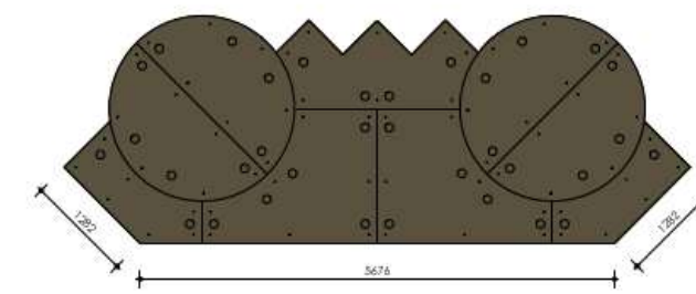
podiumdelen gekoppeld 1:50
