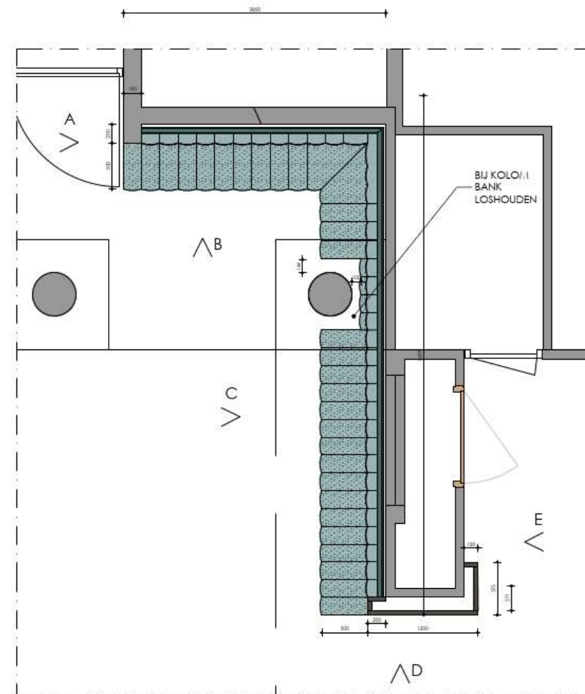
BOVENAANZICHT HOEK BANK 1:20
