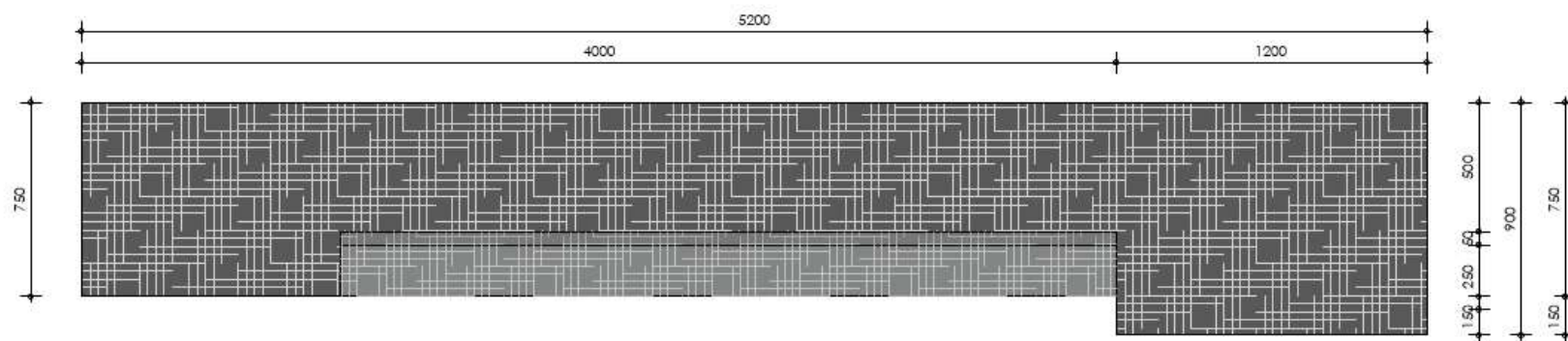
bovenaanzicht lange bank 1:20
