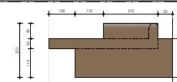
zijaaanzicht blad 1:5
