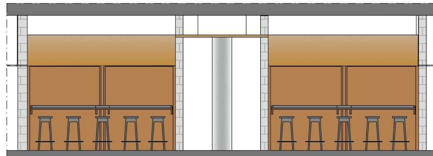
aanzicht barbladen in nissen 1:20
