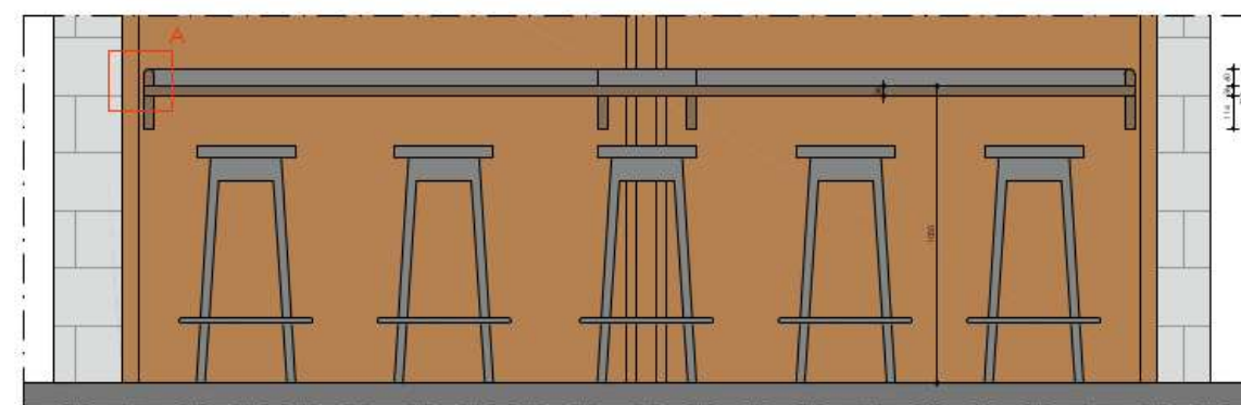
vooraanzicht blad 1:10
