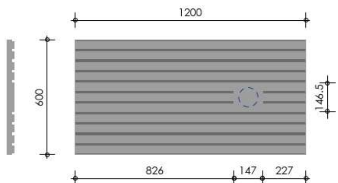
E special E - spot opliggend zijkant 1200 x 600 Troldekt® line
