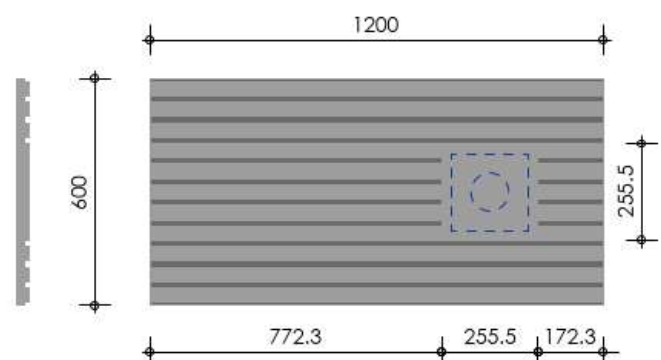
K special K - opliggend vlak groot - zijkant tbv spot / rookmelder / speaker / ... 1200 x 600 Troldekt® line
