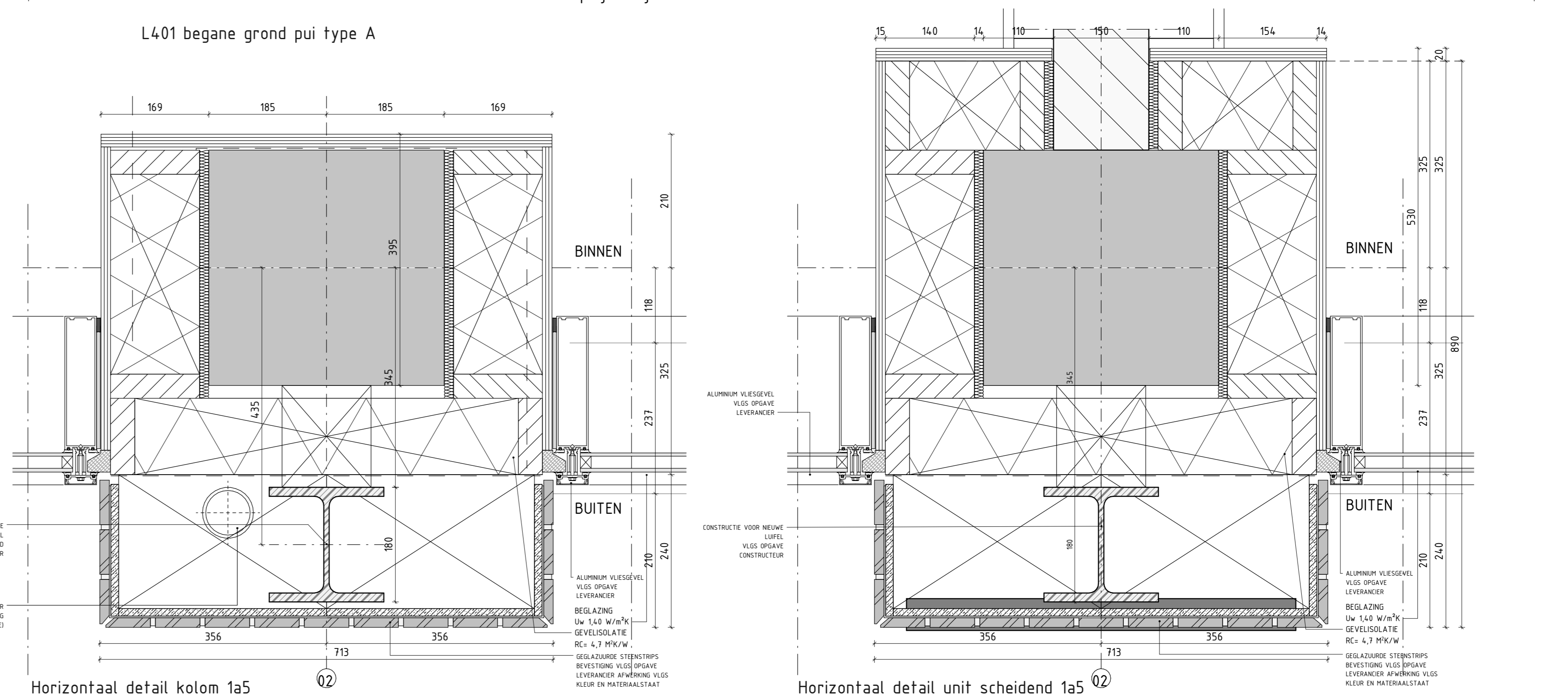
Horizontaal detail kolom 1a5
