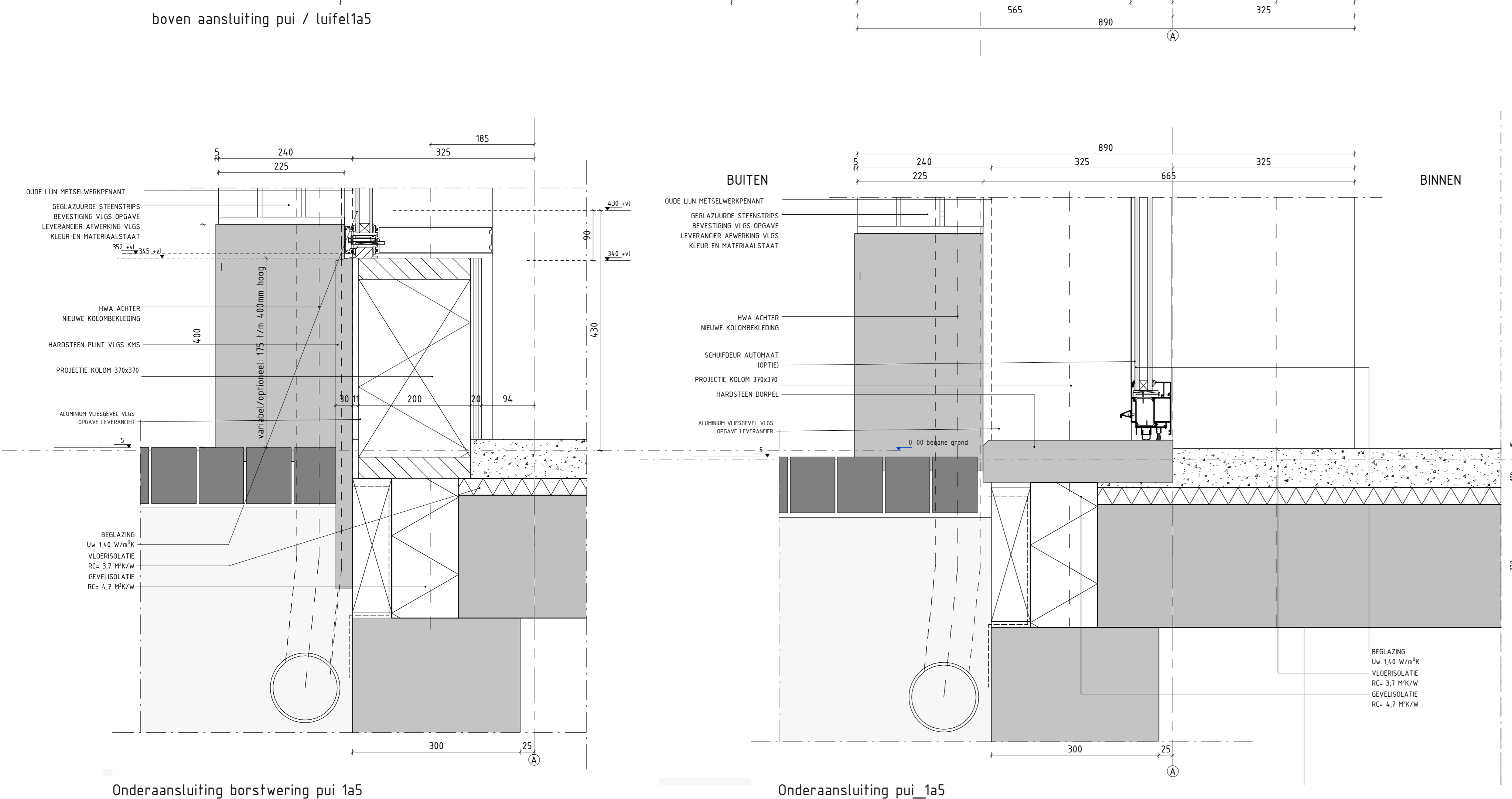
Onderaansluiting borstwing pui 1a5
