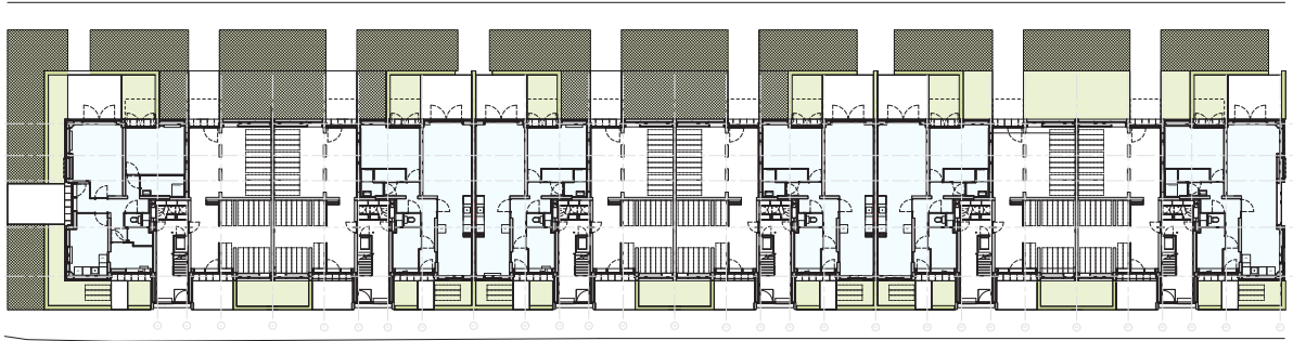
plattegrond begane grond na renovatie
