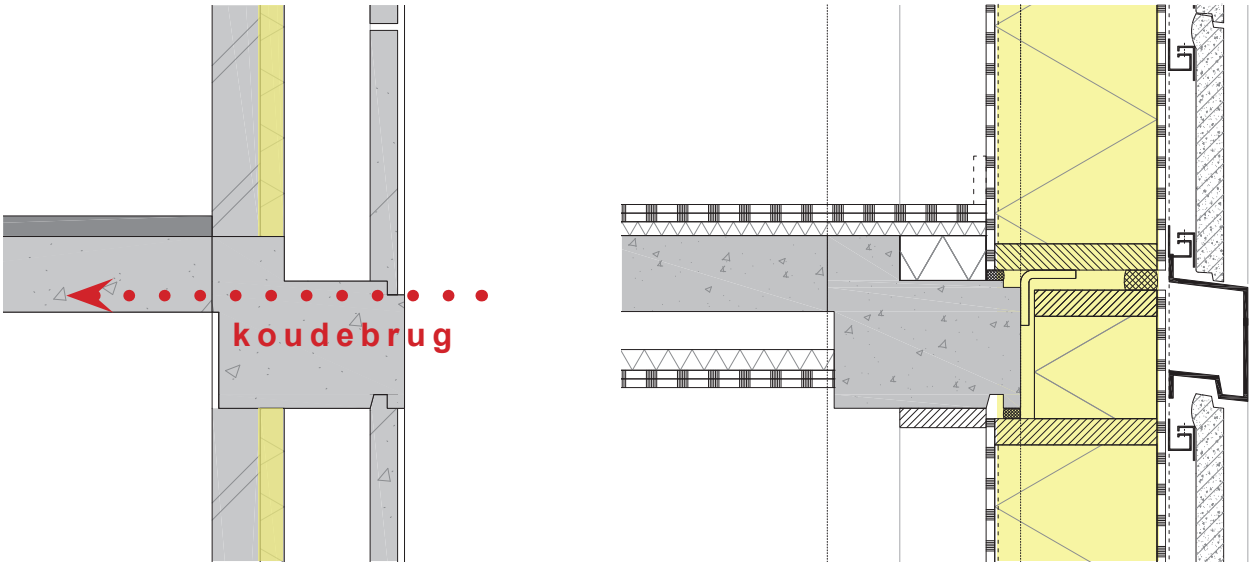
oorspronkelijk vloerranddetail (links) en vloerranddetail na renovatie (rechts)
