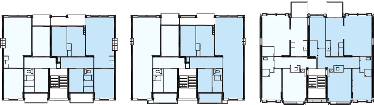
1963 1993 2023 typische woningplattegrond driekamerwoning (links) en vierkamerwoning (rechts)
