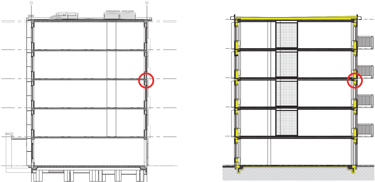
oorspronkelijke doorsnede (links) en doorsnede na renovatie (rechts)
