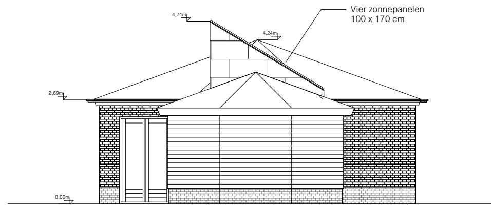
ZIJGEVEL
