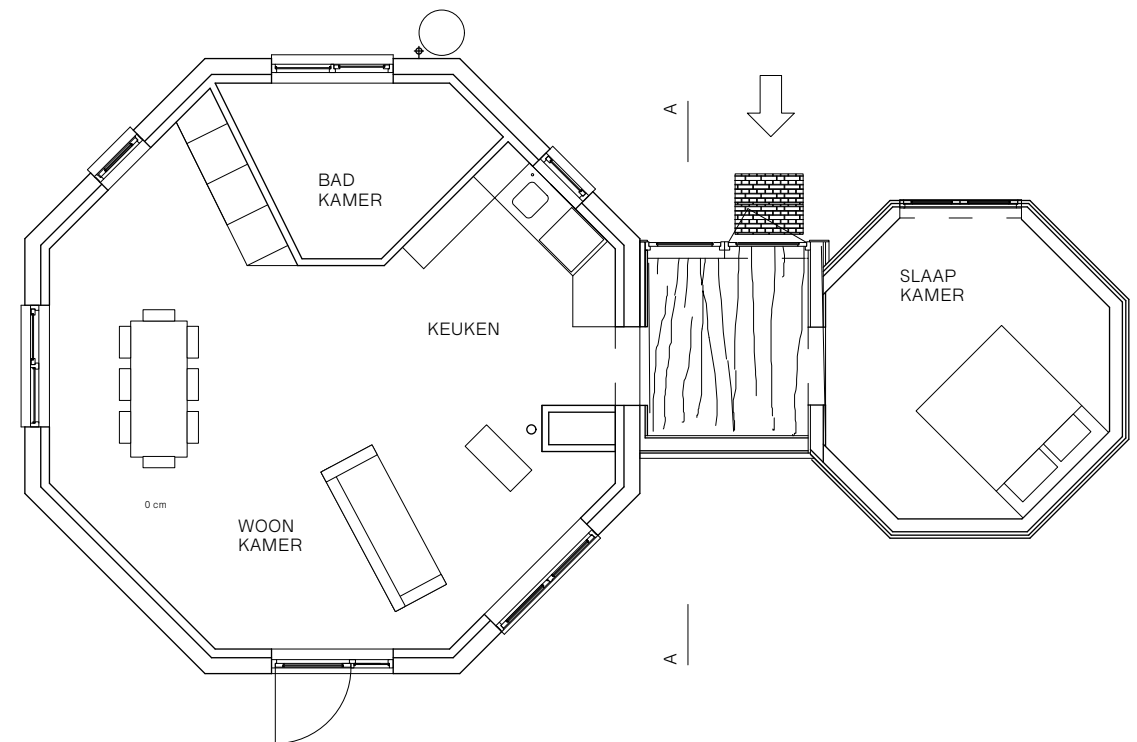
PLATTEGROND
