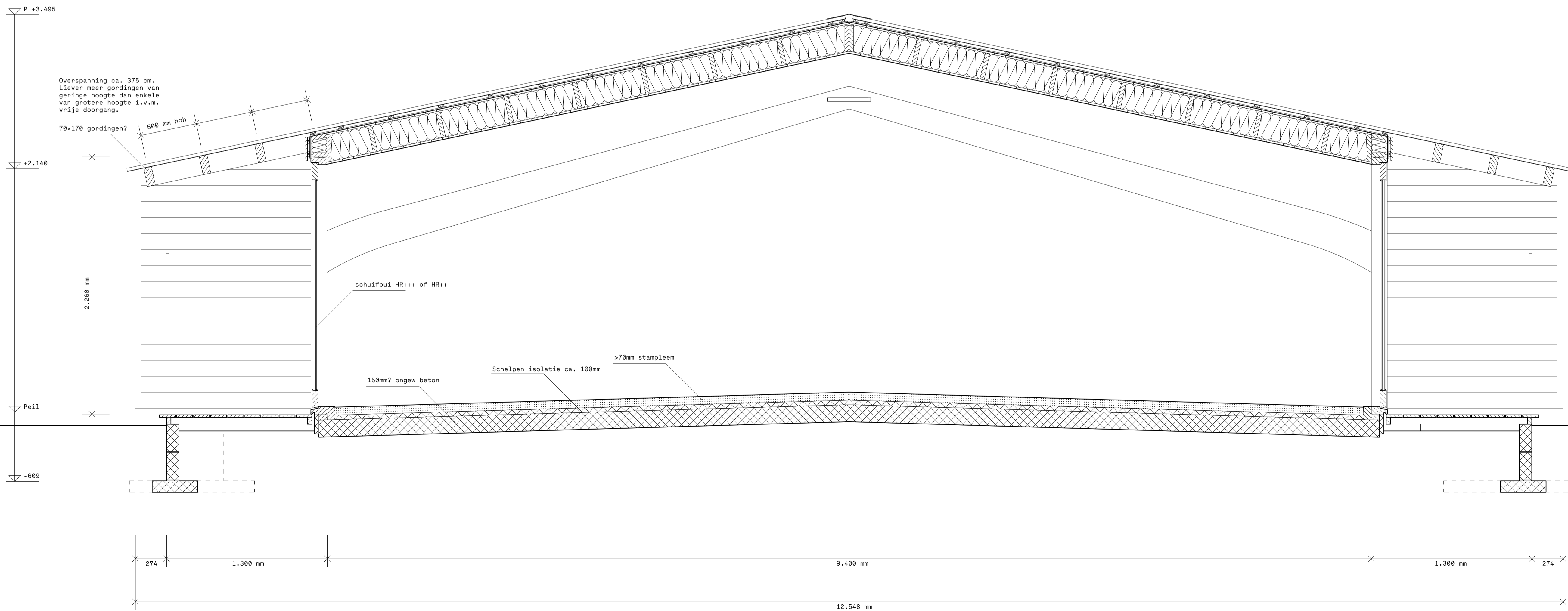
DOORSNEDE D-D
