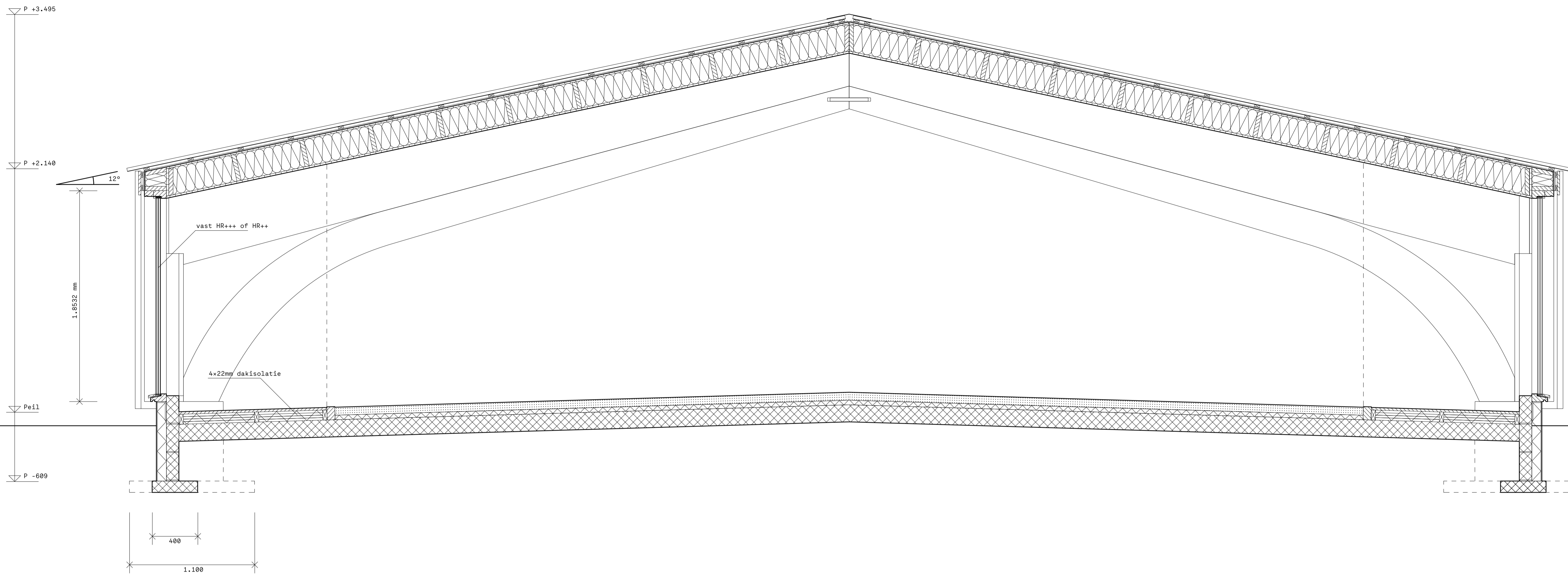
DOORSNEDE C-C
