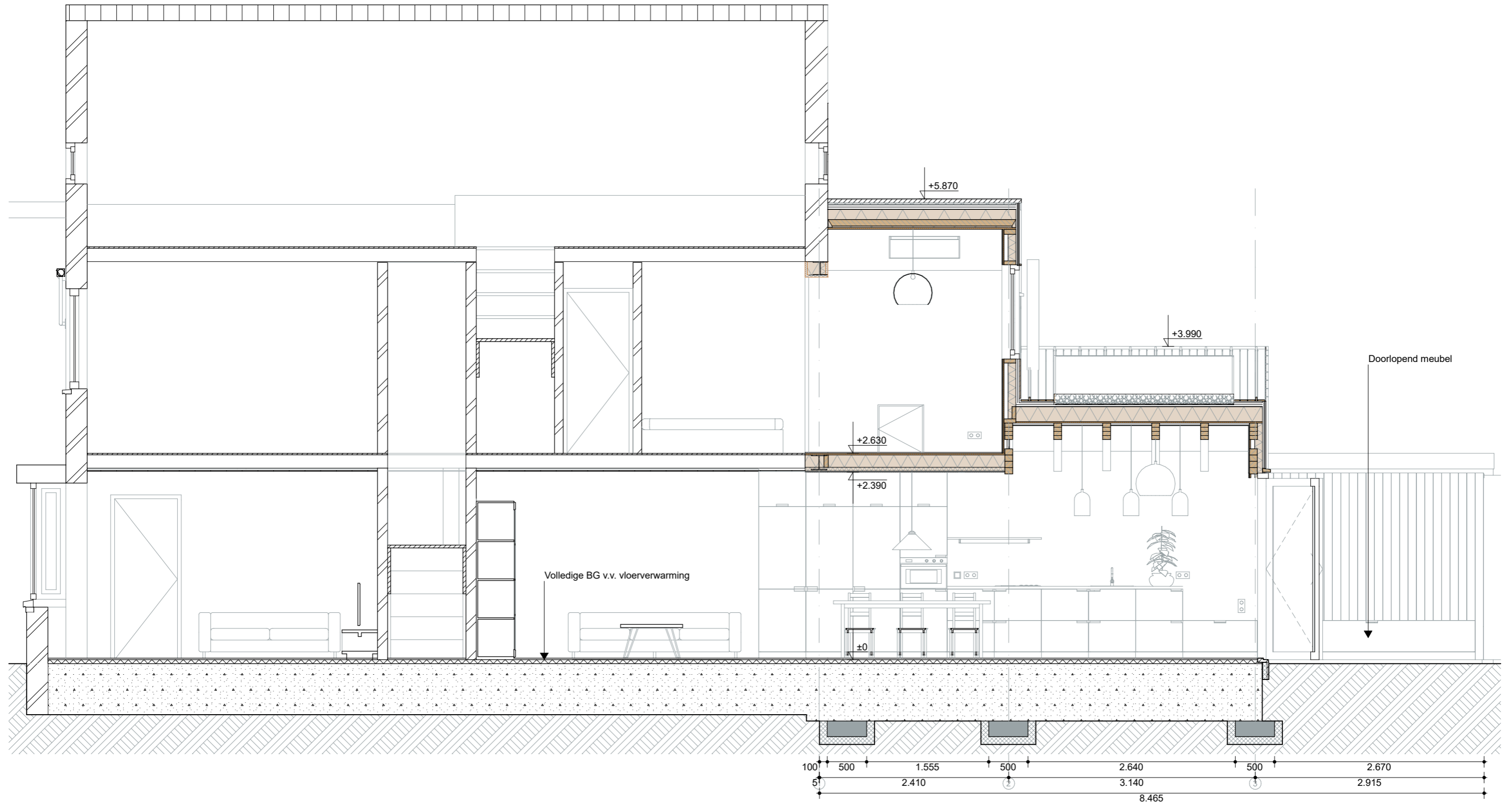
Langsdoorsnede A - nieuw - 1:50
