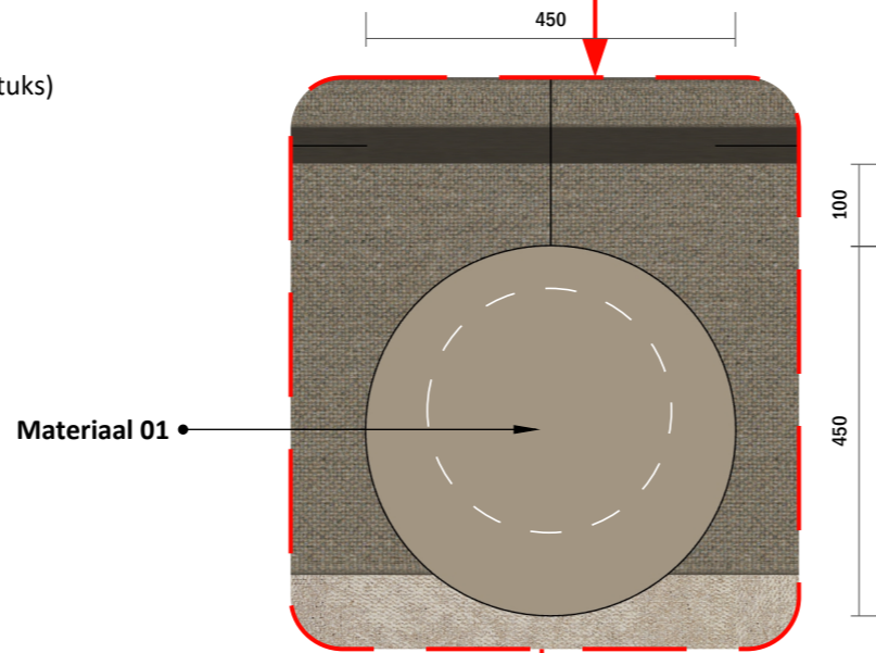
SCHAAL 1:10 (BOVENAANZICHT)
