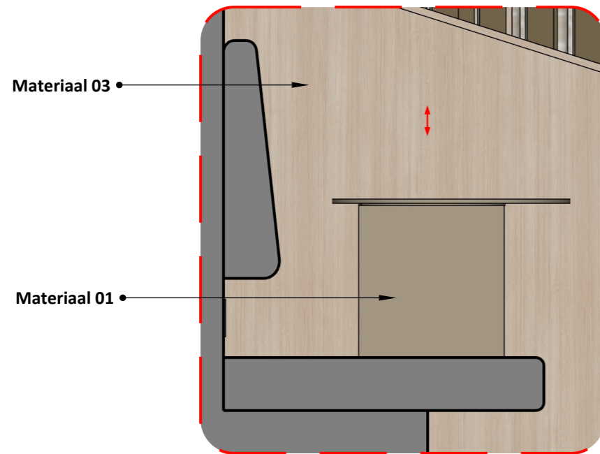
8X RONDE TAFEL, SCHAAL 1:10 (ZIJAANZICHT)
