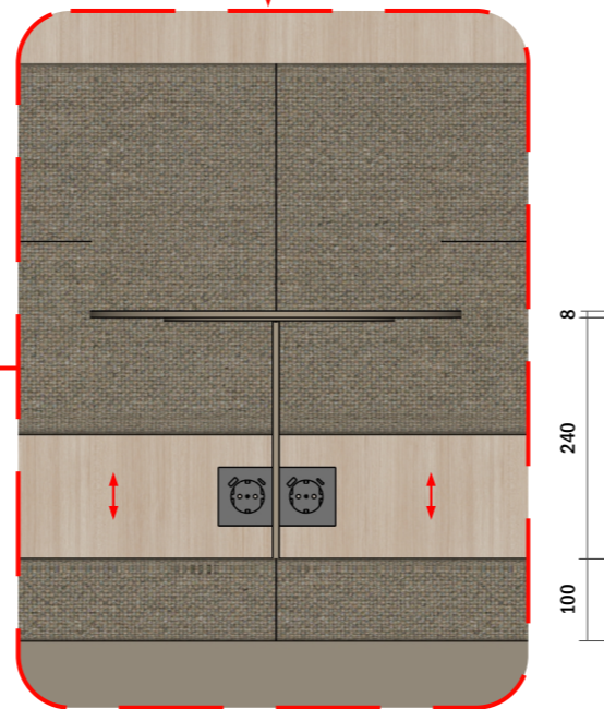
SCHAAL 1:10 (VOORAANZICHT)
