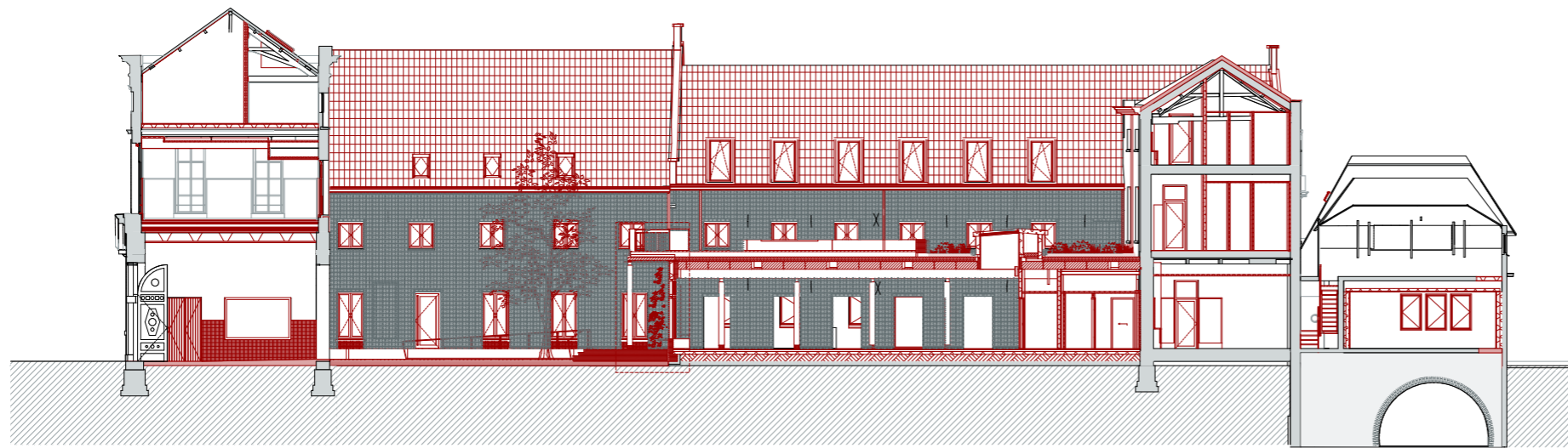
Doorsnede C
