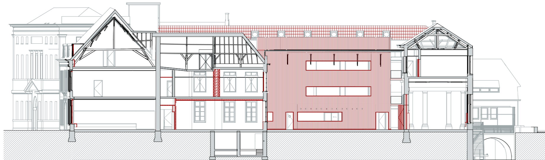
Doorsnede D
