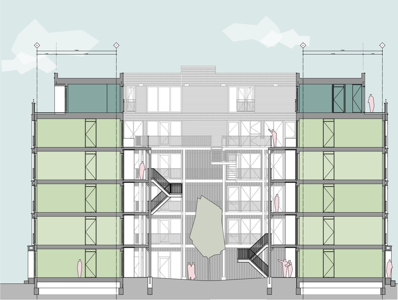
DOORSNEDE B-B
