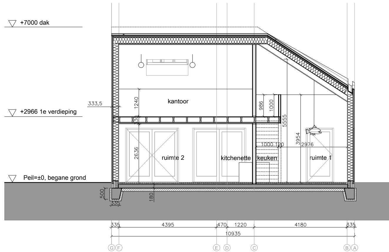
doorsnede CC'
