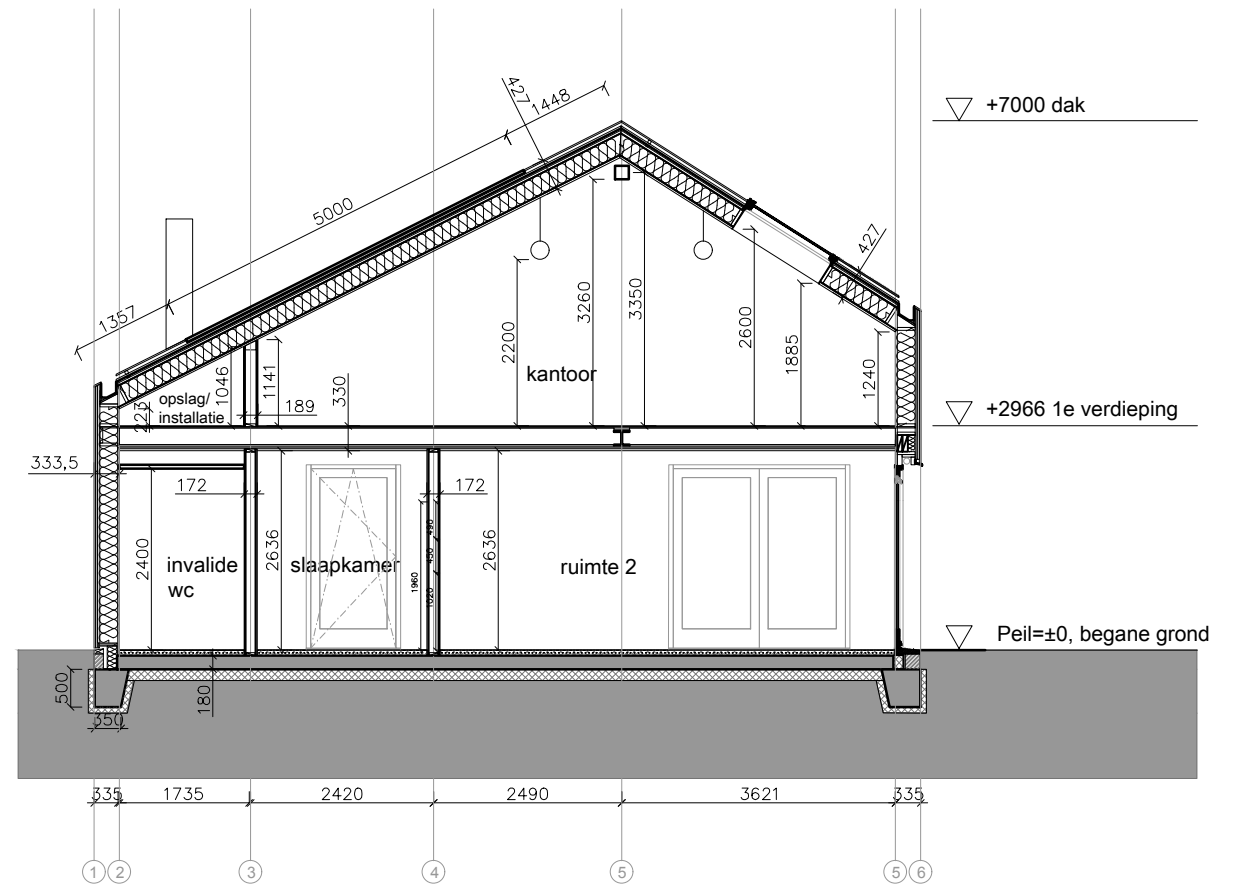
doorsnede BB'
