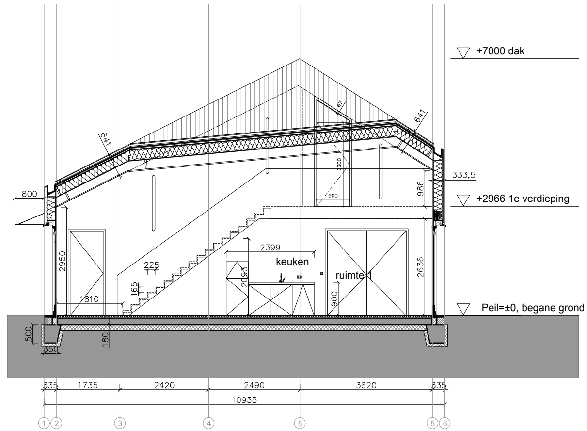
doorsnede AA'
