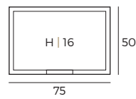
Klein - S
