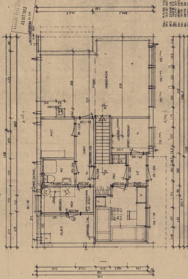
PLAN UNDERFETASJE
