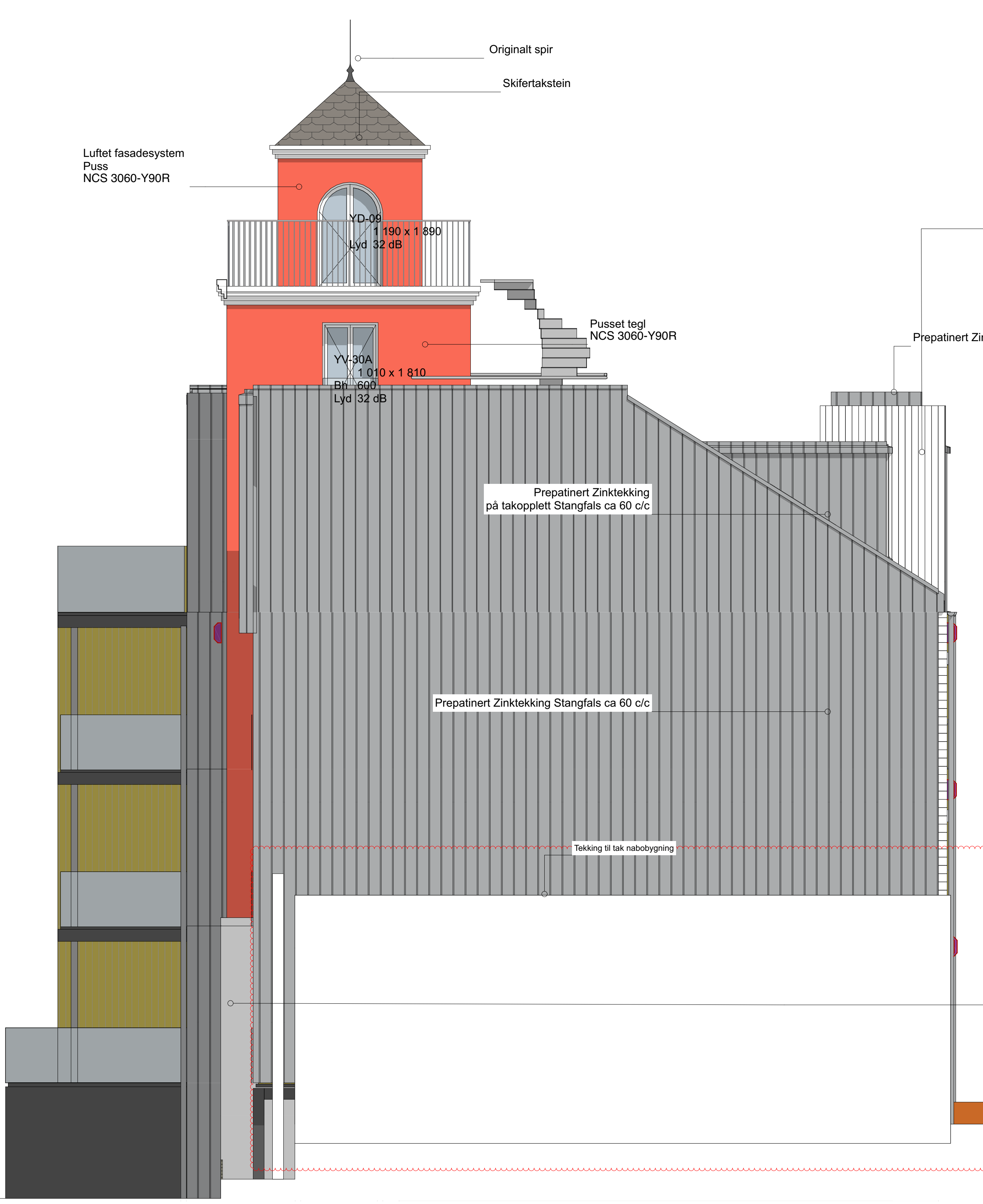
Fasade Sør 1:50
