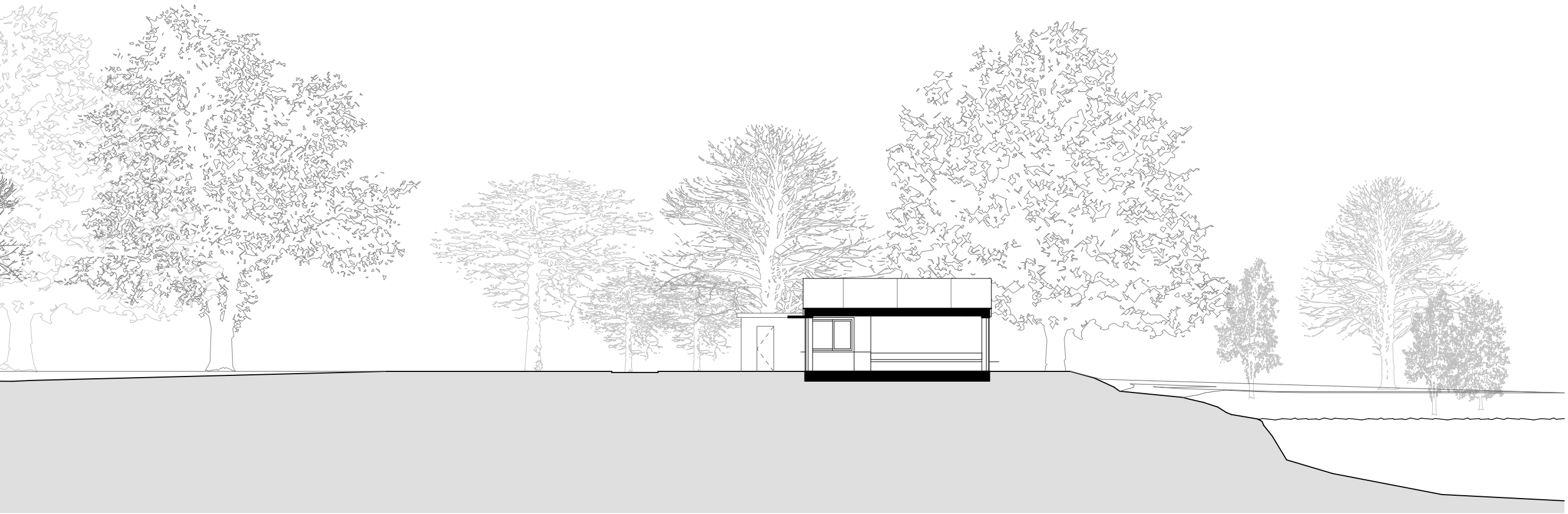
Sektion 1:200
