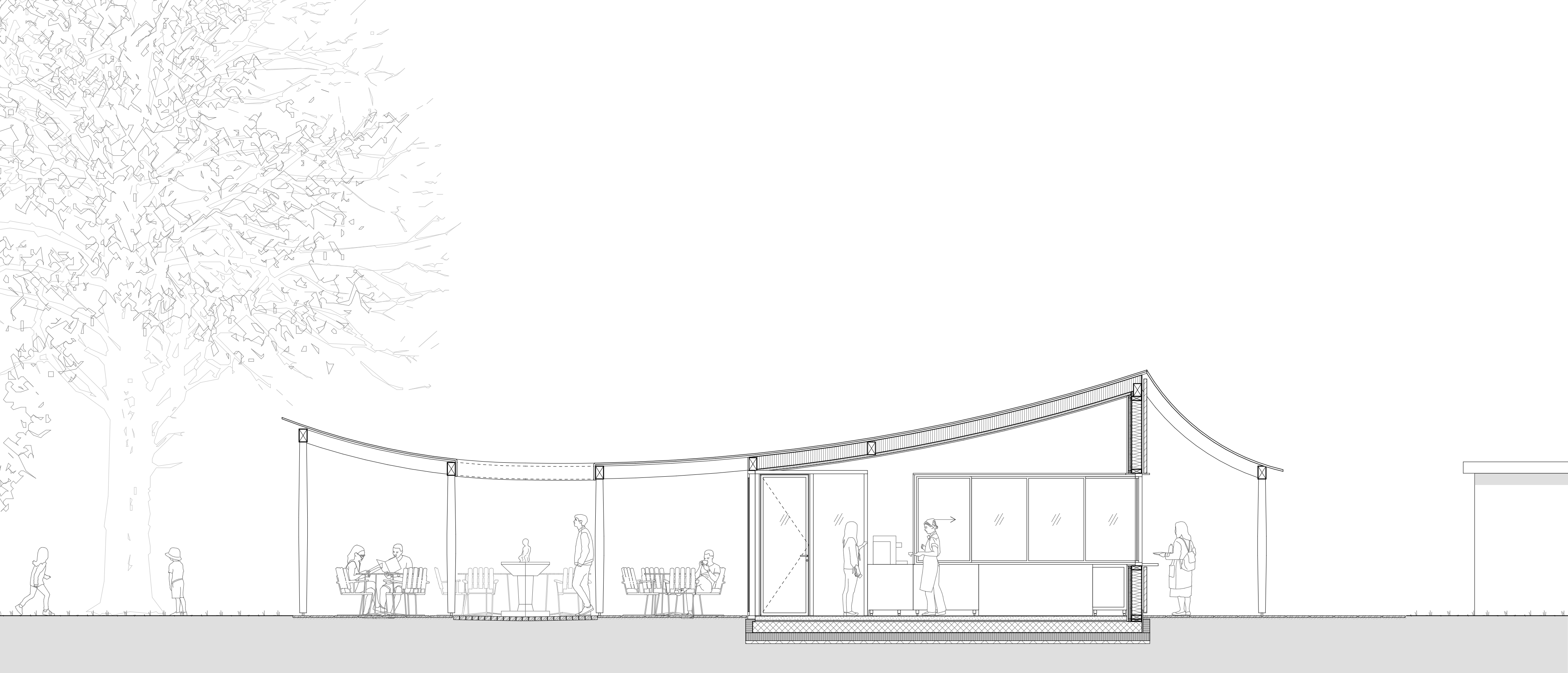
Sektion 1:50
