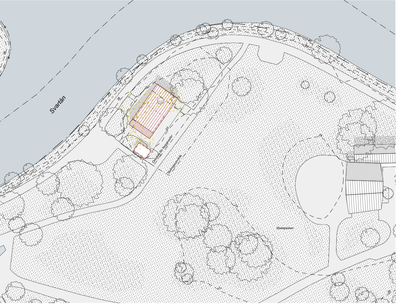
Situationsplan Rives i gult och nytt i rött. 1:800
