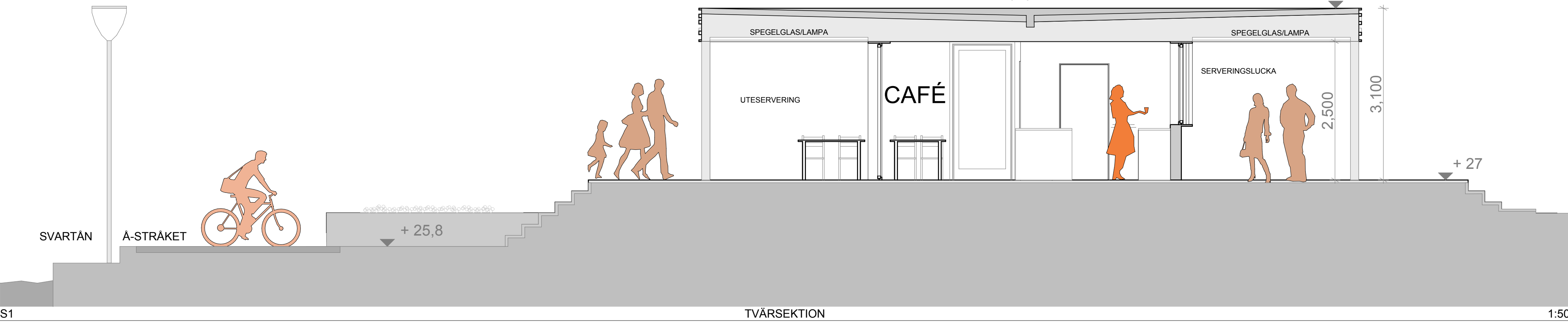
TVÄRSEKTION
