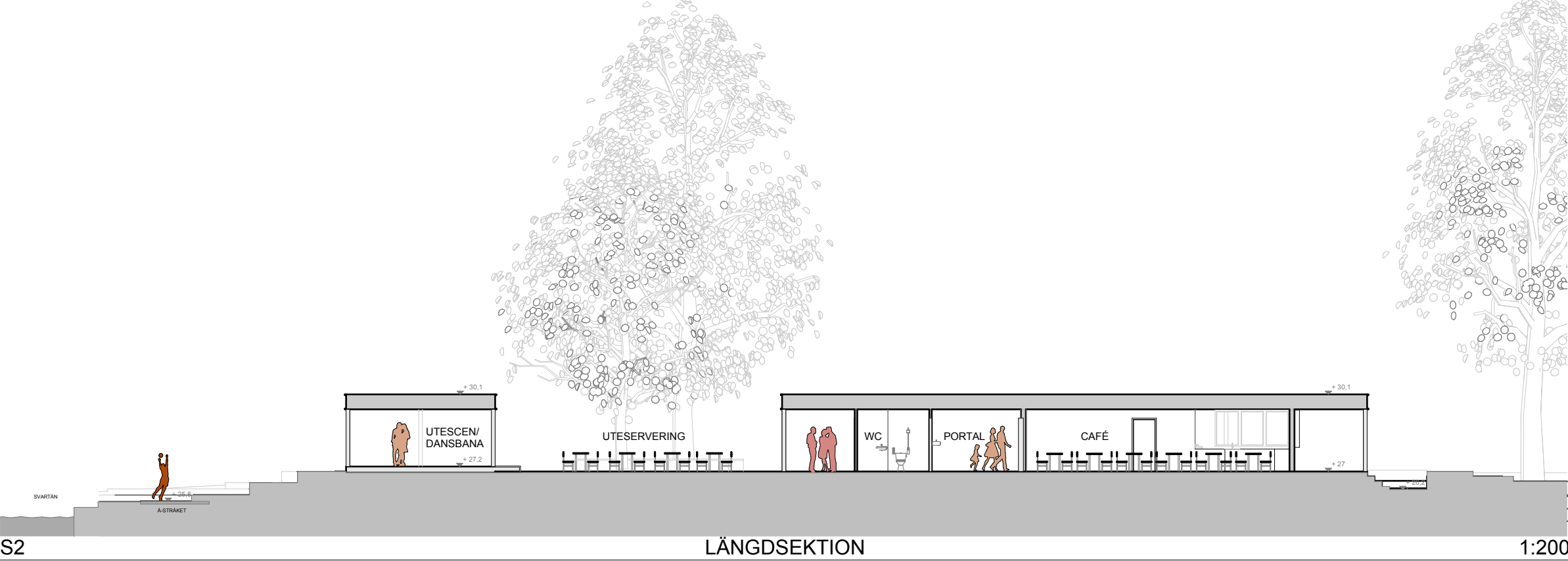
LÅNGDSEKTION
