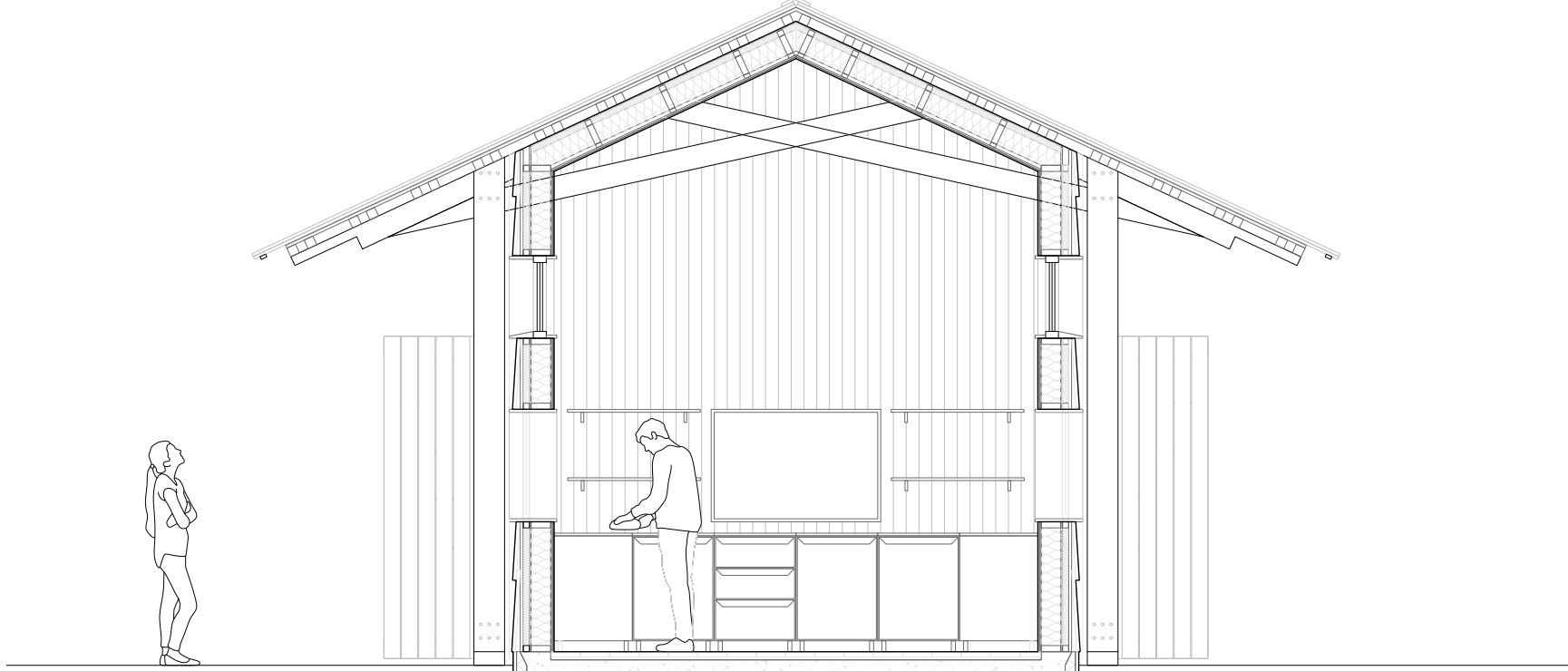
Sektion B-B Skala - 1:50 (A1)
