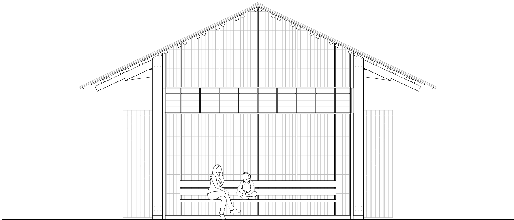
Fasad mot söder Skala - 1:50 (A1)
