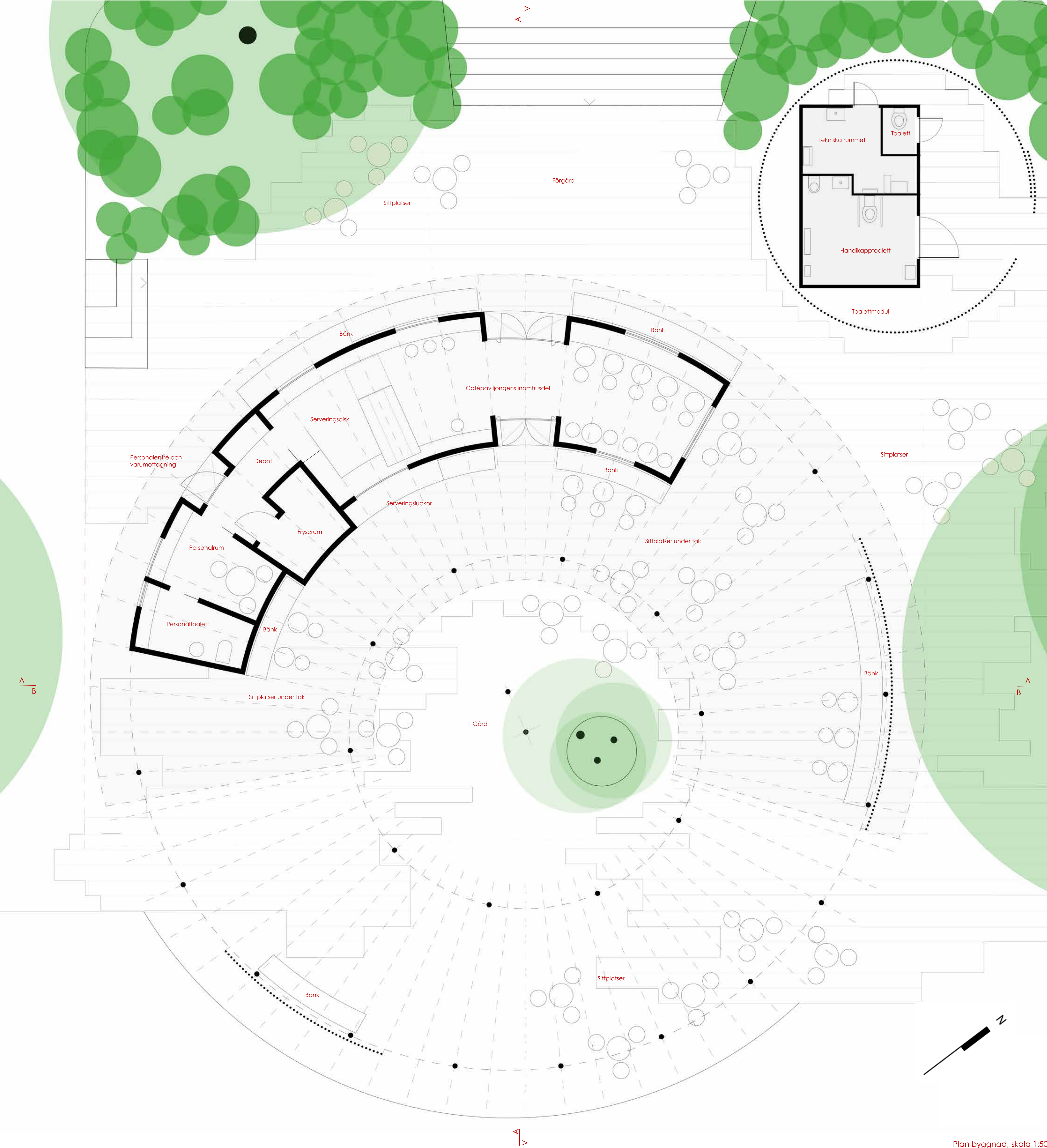
Plan byggnad, skala 1:50
