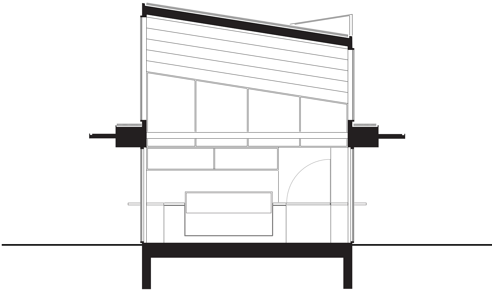
Sektion AA 1:50
