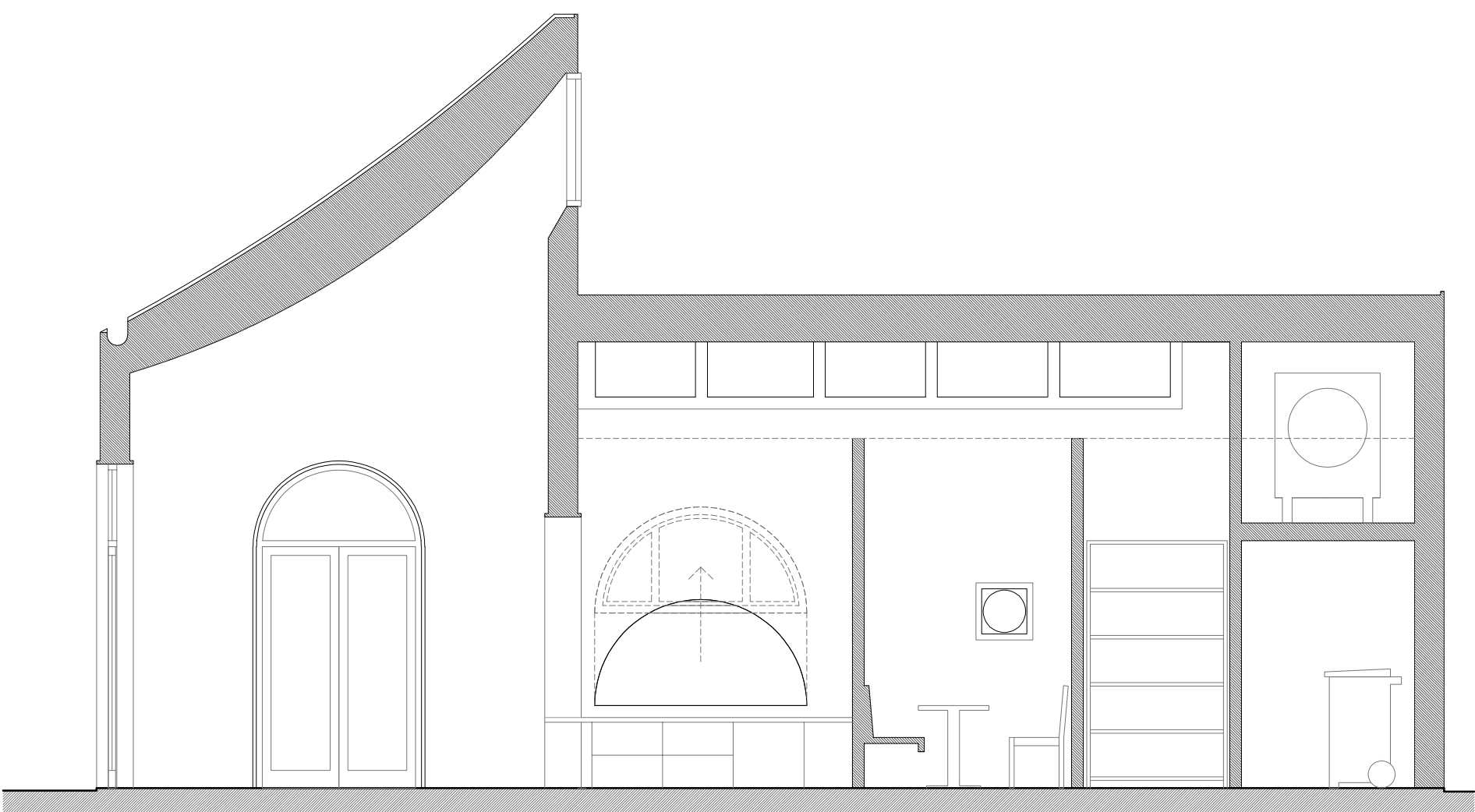
Sektion A-A Skala 1:50
