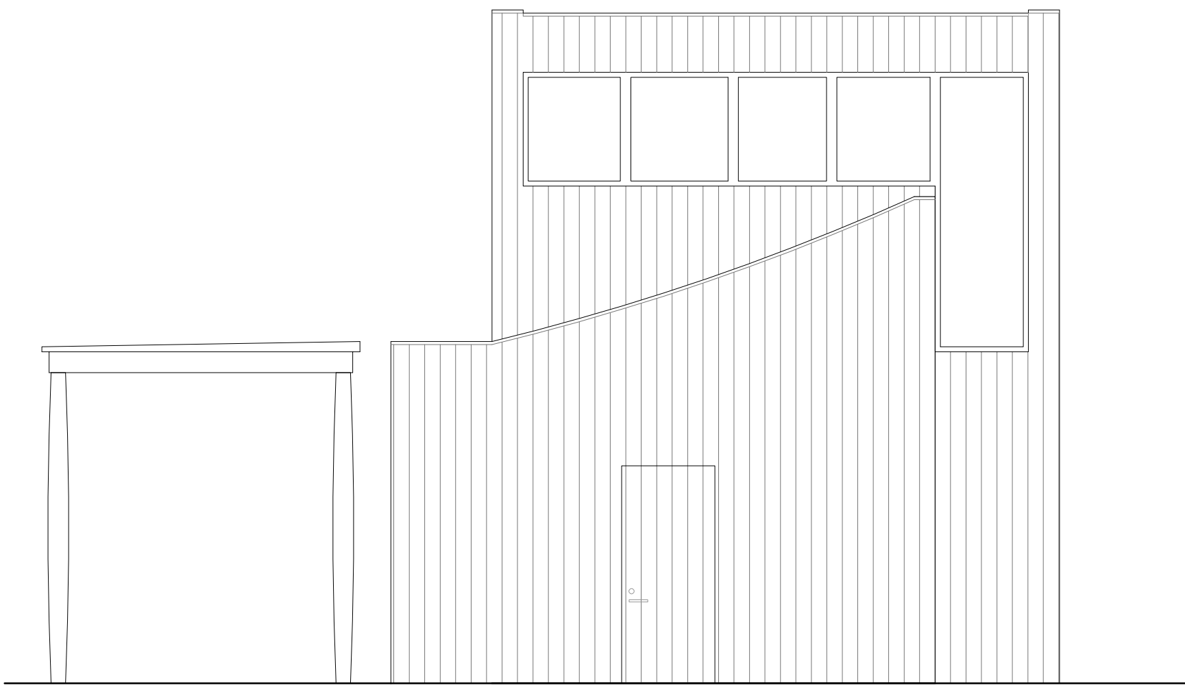
Fasad mot Nordöst Skala 1:50
