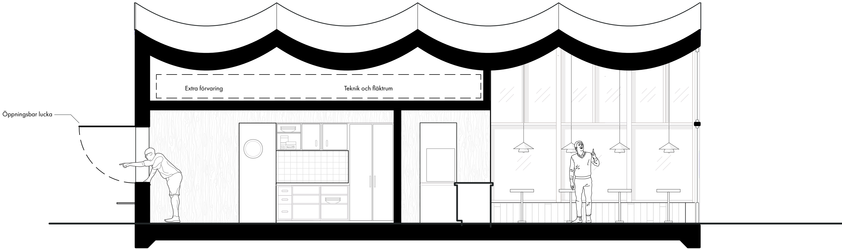
SEKTIÖN B-B (1:50) SE PLAN 1:50 FÖR DRAGNING
