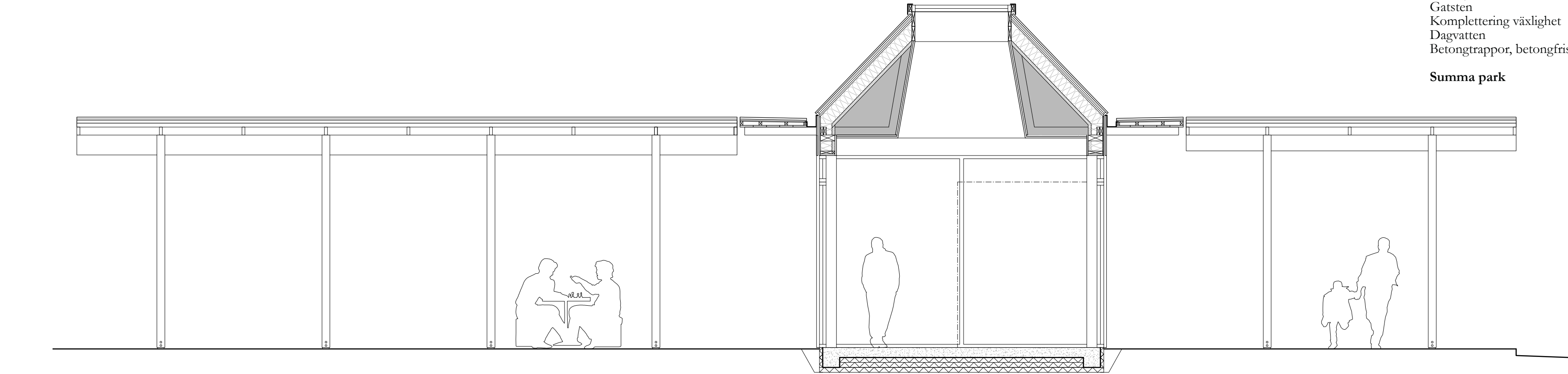
Sektion A-A, skala 1:50
